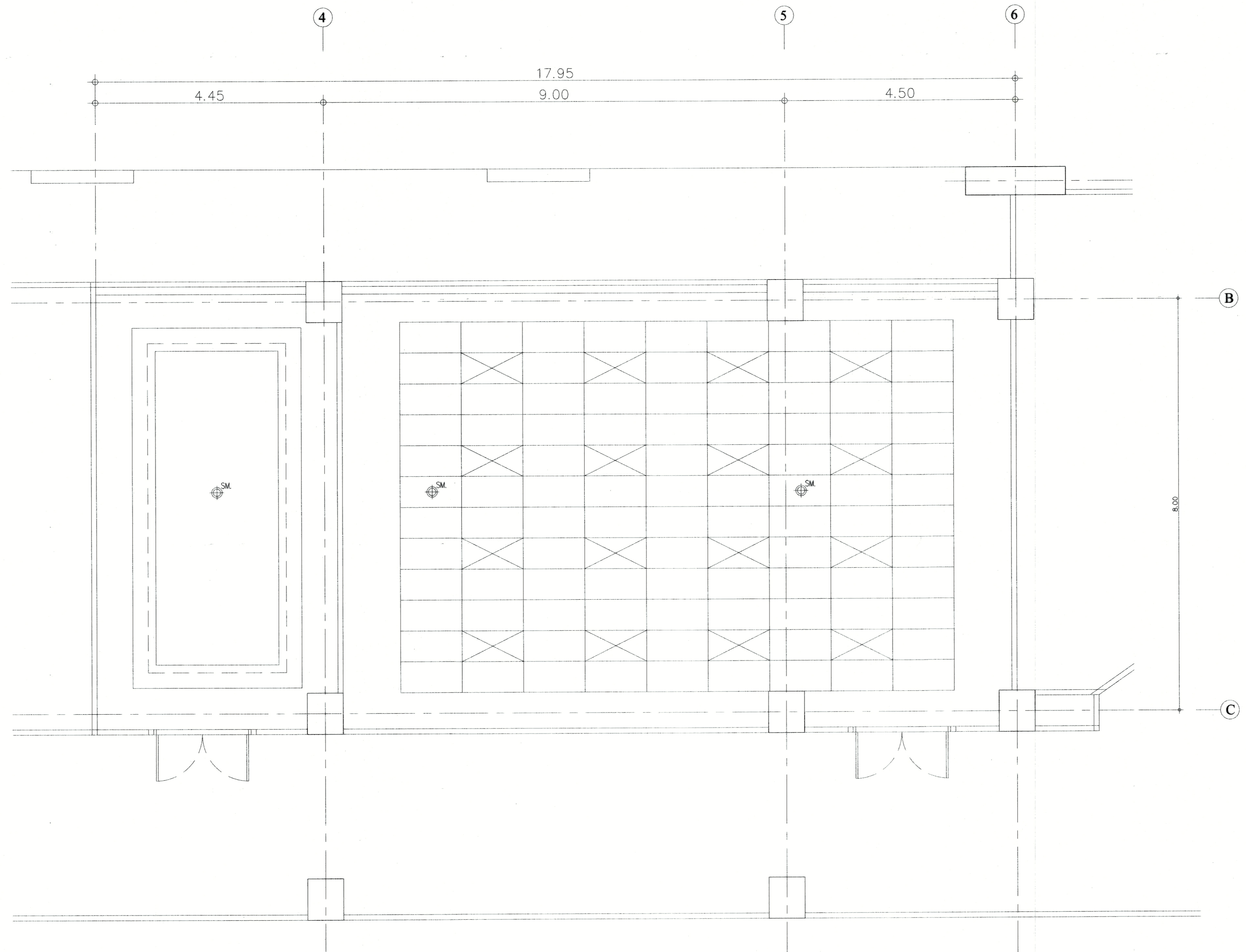
แปลน ตัวตรวจจับควันและความร้อน 150 สำนักงาน ชั้น 2 (หลังปรับปรุง)
