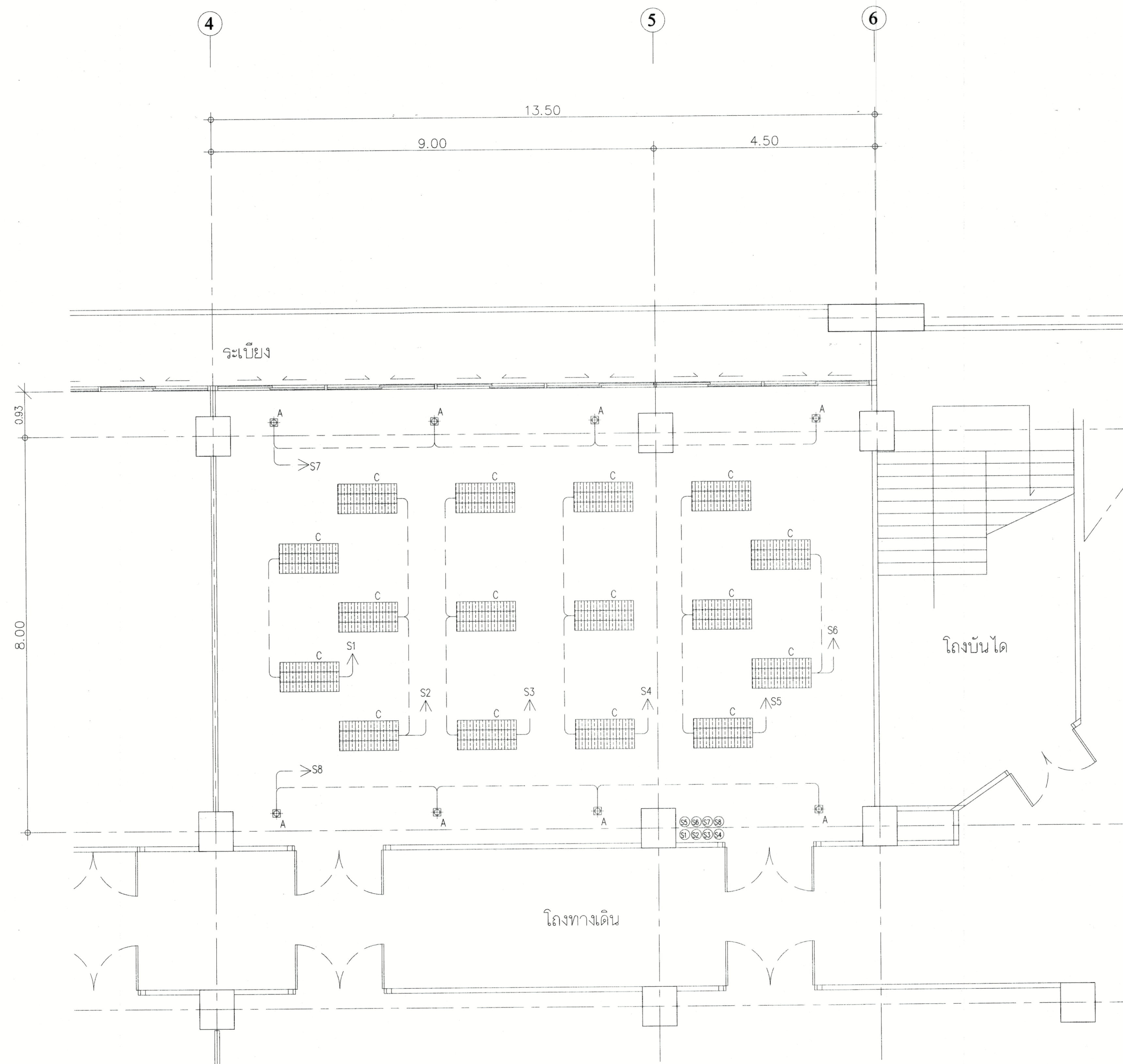
150 แปลน ไฟฟ้าแสงสว่าง ห้อง 606 , 608 ชั้น 6 (หลังปรับปรุง) ระบบไฟต่อกับตู้คอนโทรลลิ้ม ไฟพร้อมใช้งาน
