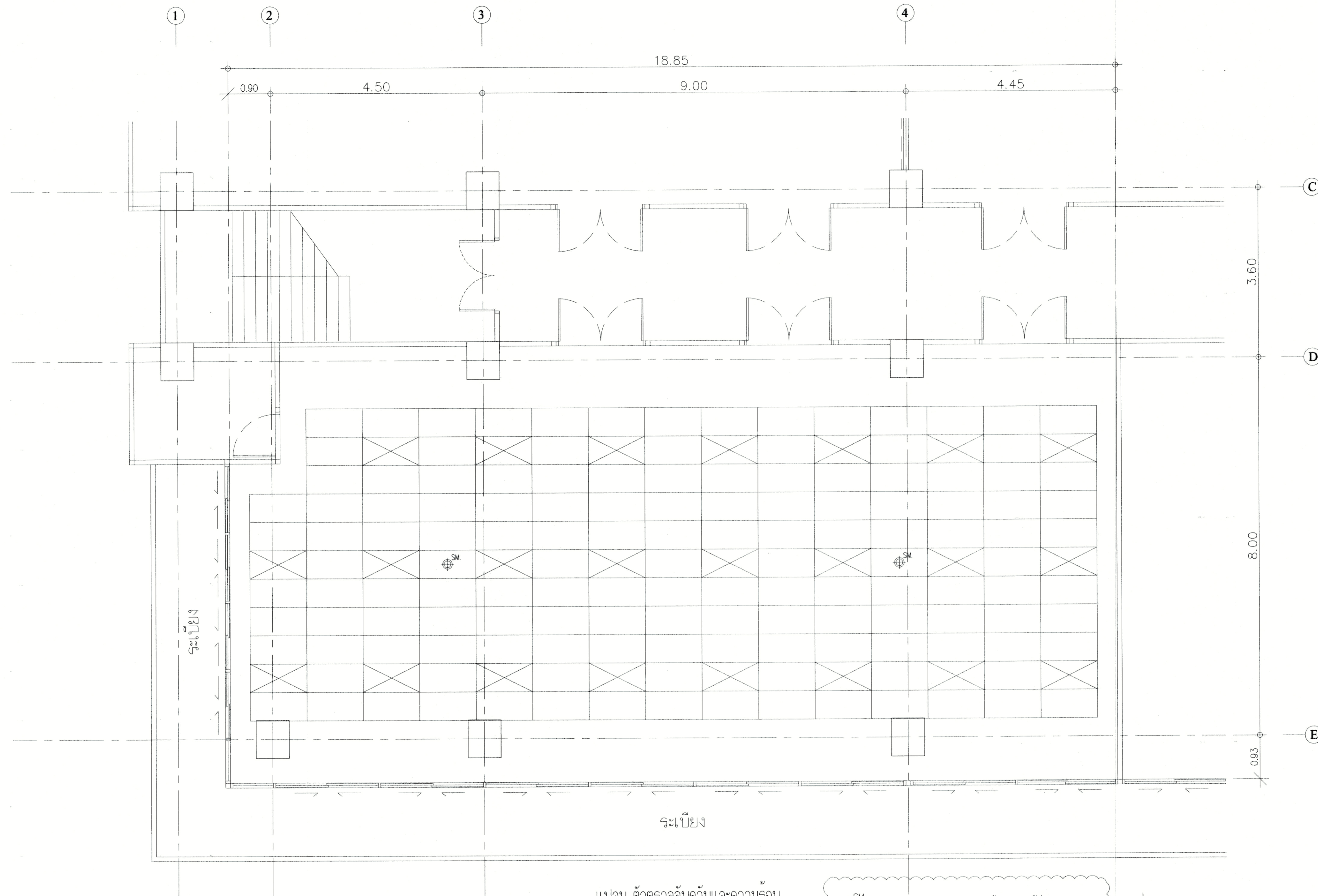
แปลน ตัวตรวจจับควันและความร้อน ห้อง 501 ชั้น 5 (หลังปรับปรุง)
