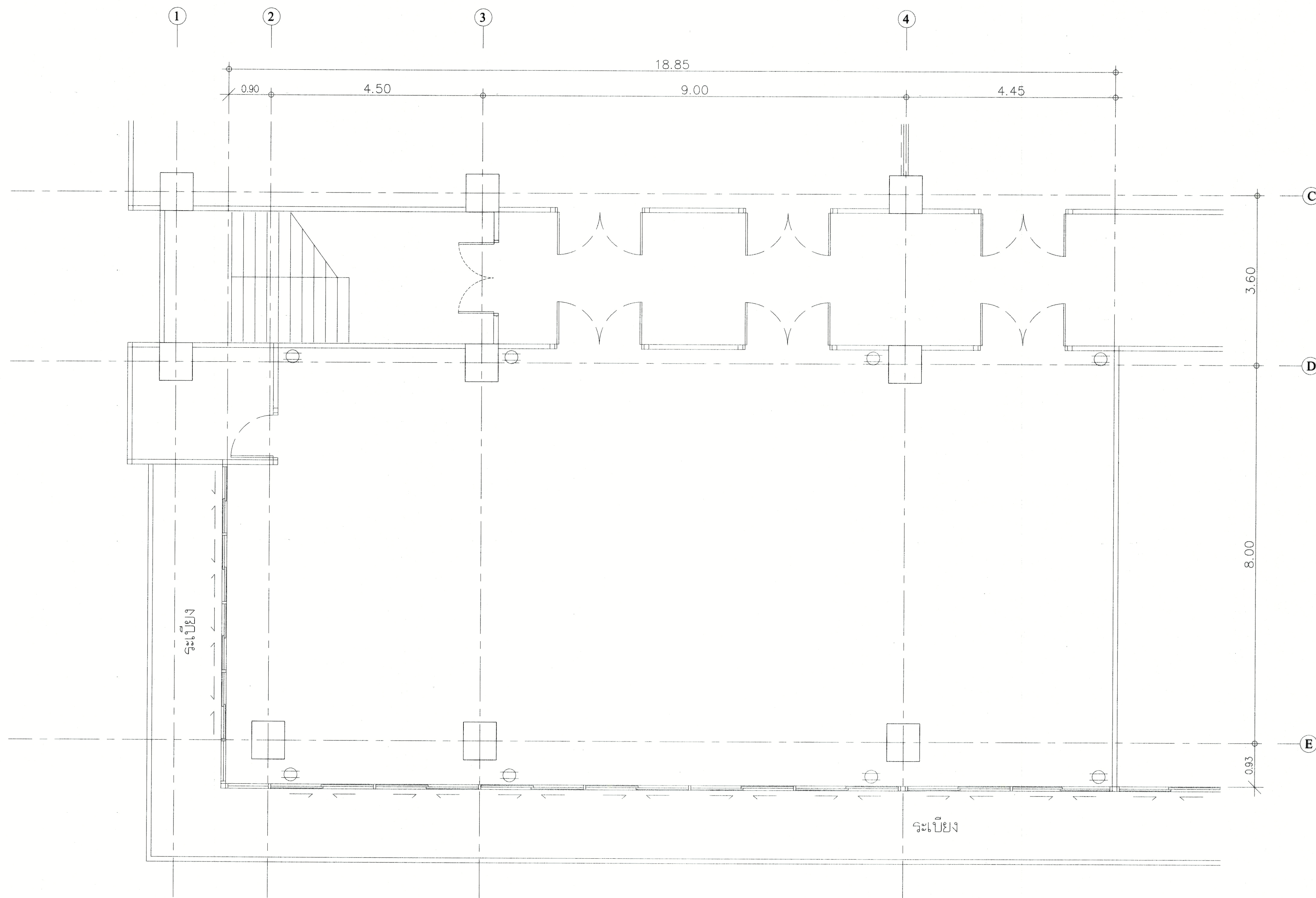
แปลน เต้าเสียบ ห้อง 501 ชั้น 5 (ไม่รวม) 1:50 (หลังปรับปรุง) ระบบไฟฟ้ากับตู้คอนโทรลเดิม ให้พร้อมใช้งาน
