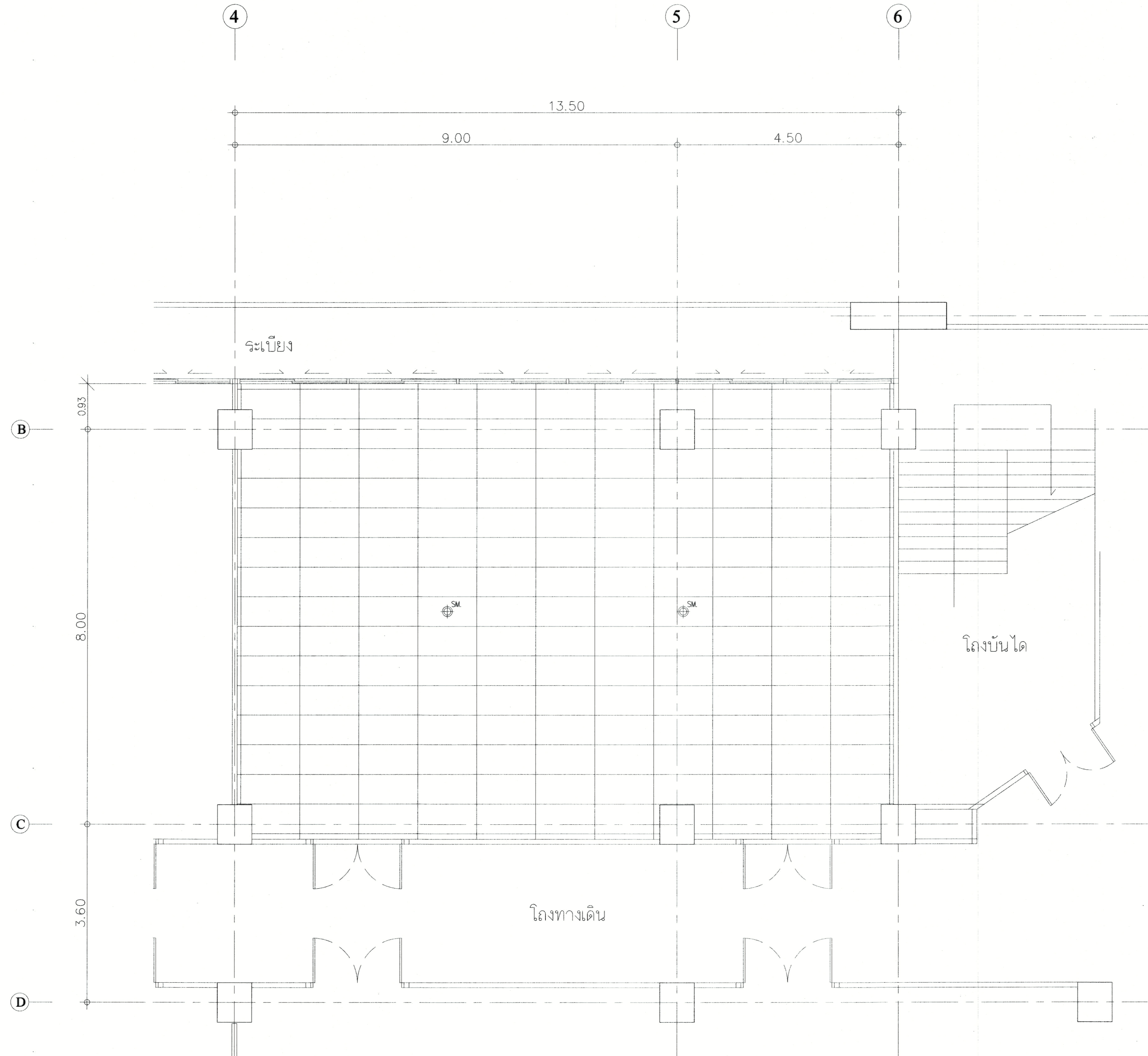
แปลน ตัวตรวจจับควันและความร้อน ห้อง 606 , 608 ชั้น 6 (ก่อนปรับปรุง)
