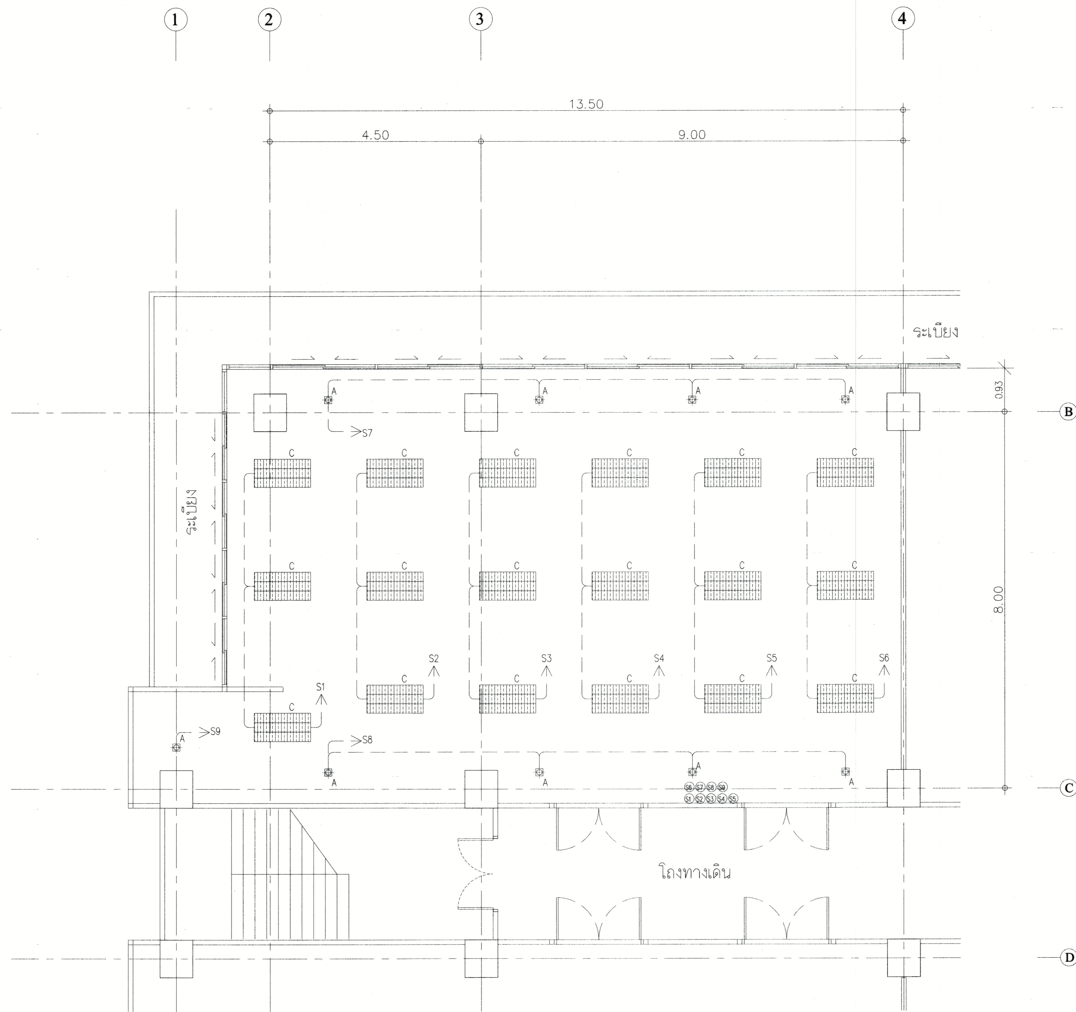
แปลน ไฟฟ้าแสงสว่าง ห้อง 602 , 604 ชั้น 6 (หลังปรับปรุง) ระบบไฟต่อกับตู้คอนโทรลเดิม ไฟพร้อมใช้งาน
