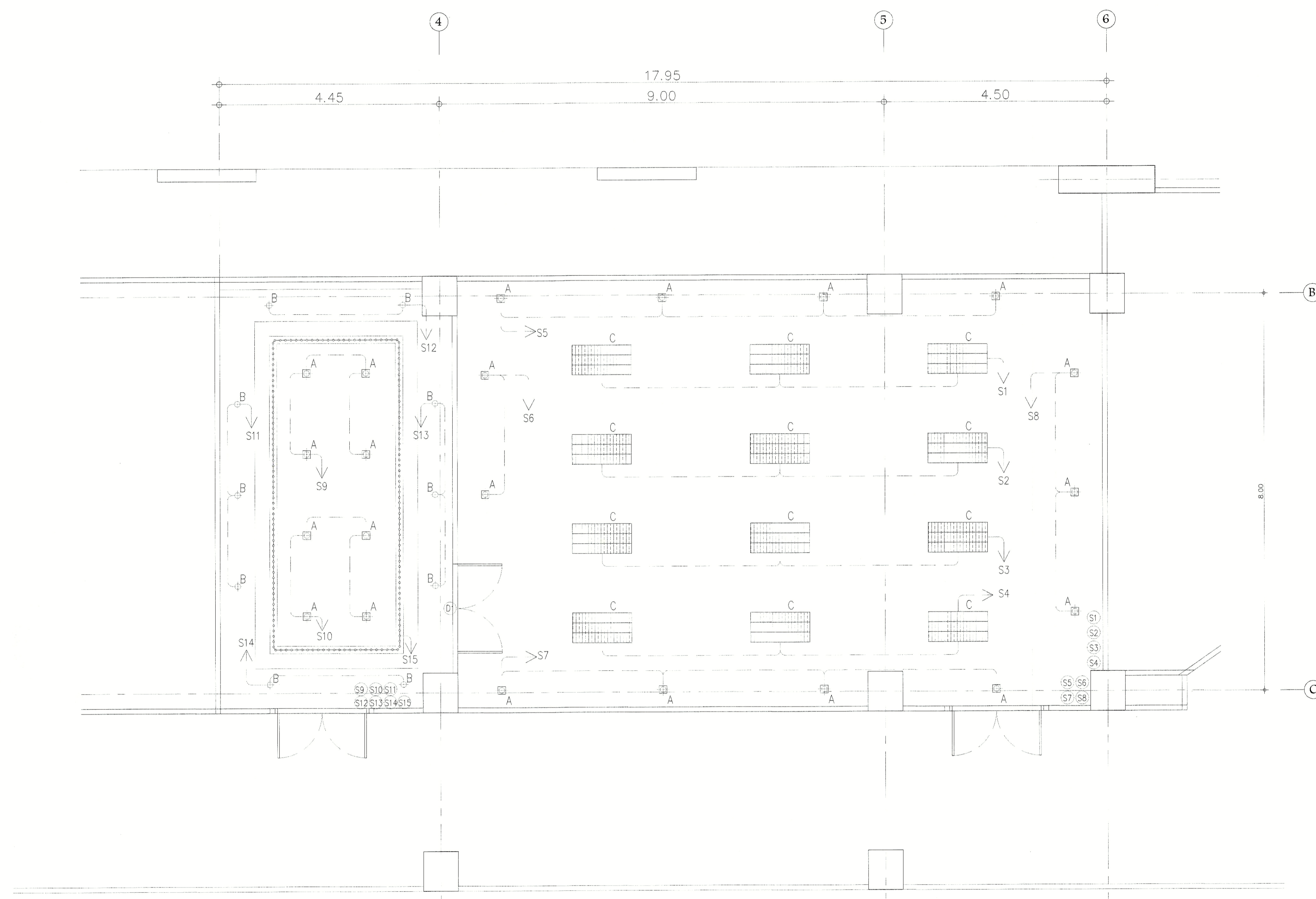
แปลน ไฟฟ้าแสงสว่าง สำนักงาน ชั้น 2 (หลังปรับปรุง) ระบบไฟต่อกับตู้คอนโทรลเดิม ให้อบรมใช้งาน
