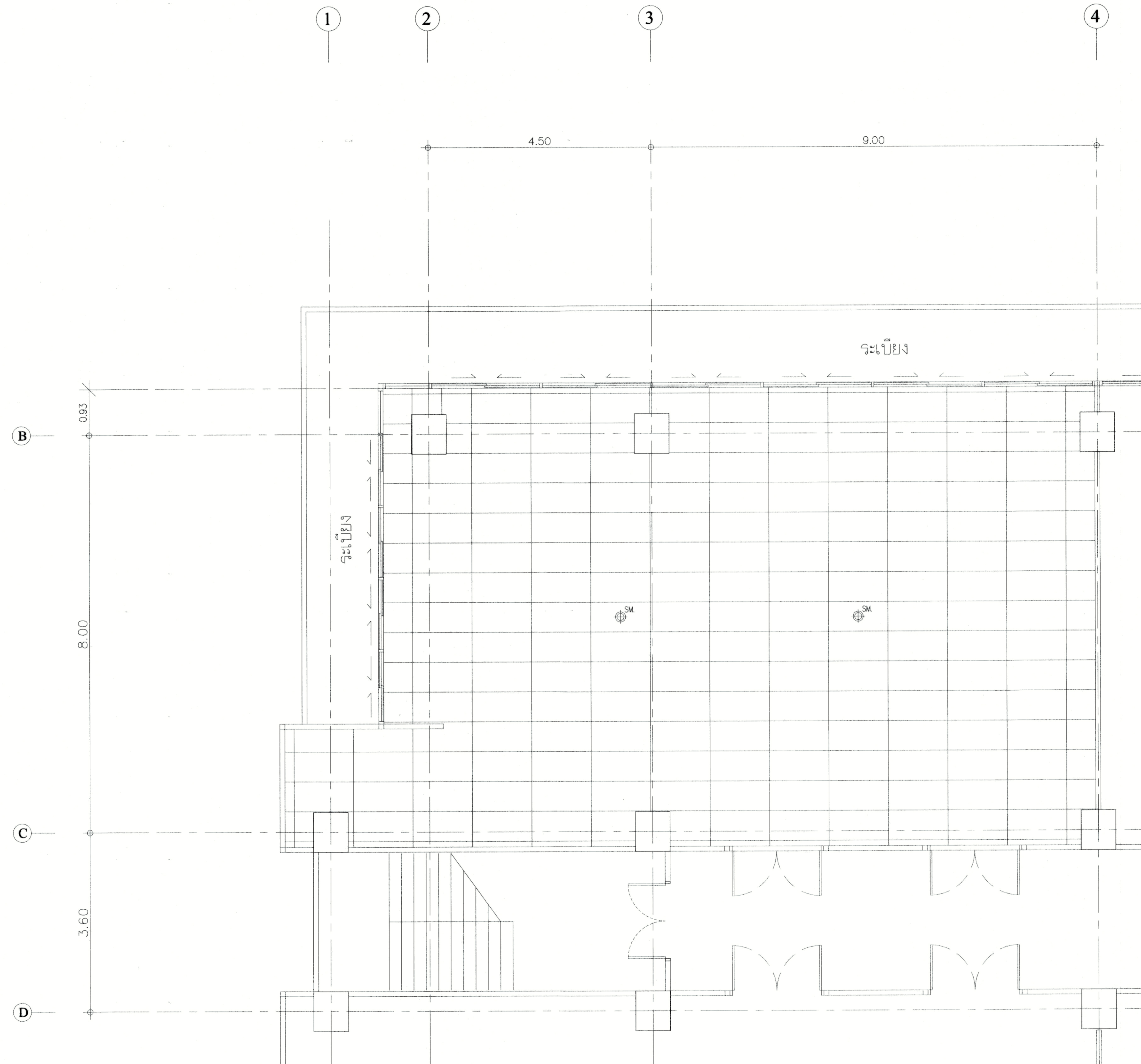
แปลน ตัวตรวจจับควันและความร้อน ห้อง 802 , 804 ชั้น 8 (ก่อนปรับปรุง)
