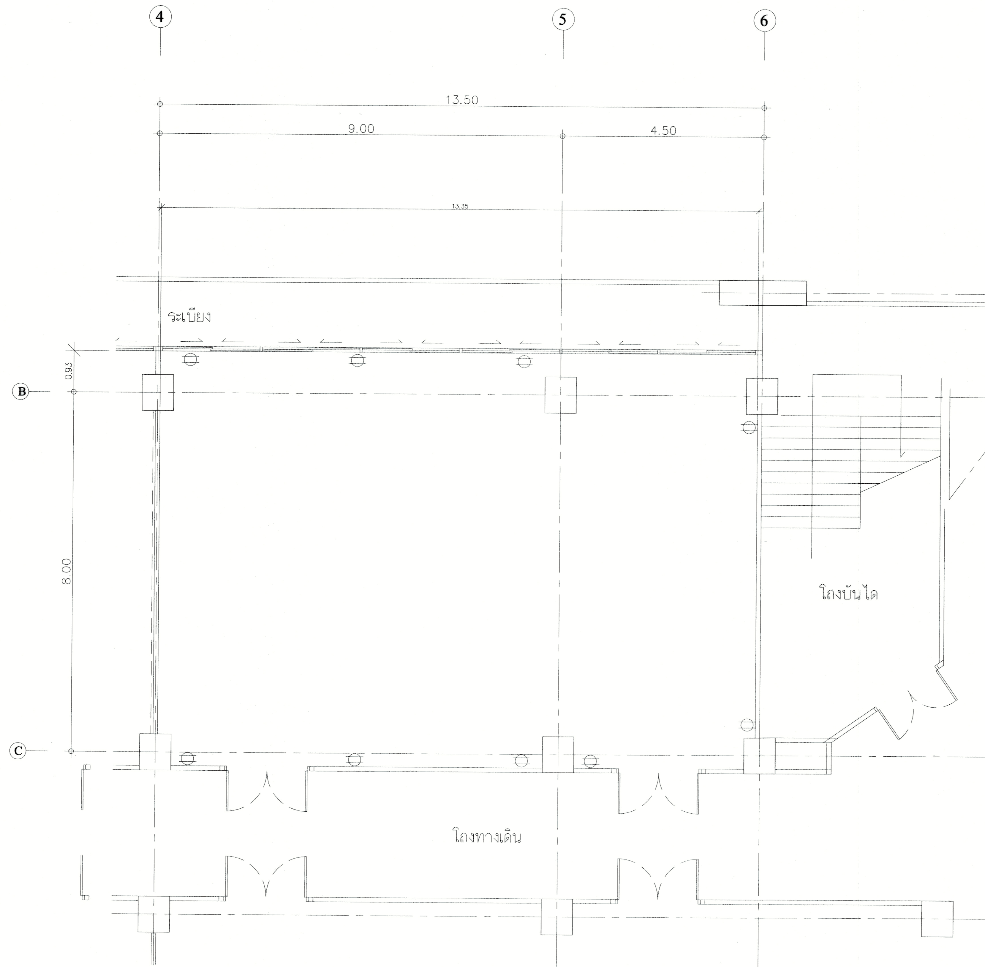
แปลน เตาเลียบ ห้อง 806 , 808 ชั้น 8 (ไม่รวม) (หลังปรับปรุง) ระบบไฟติดกับตู้คอนโทรลเดิม ให้พร้อมใช้งาน
