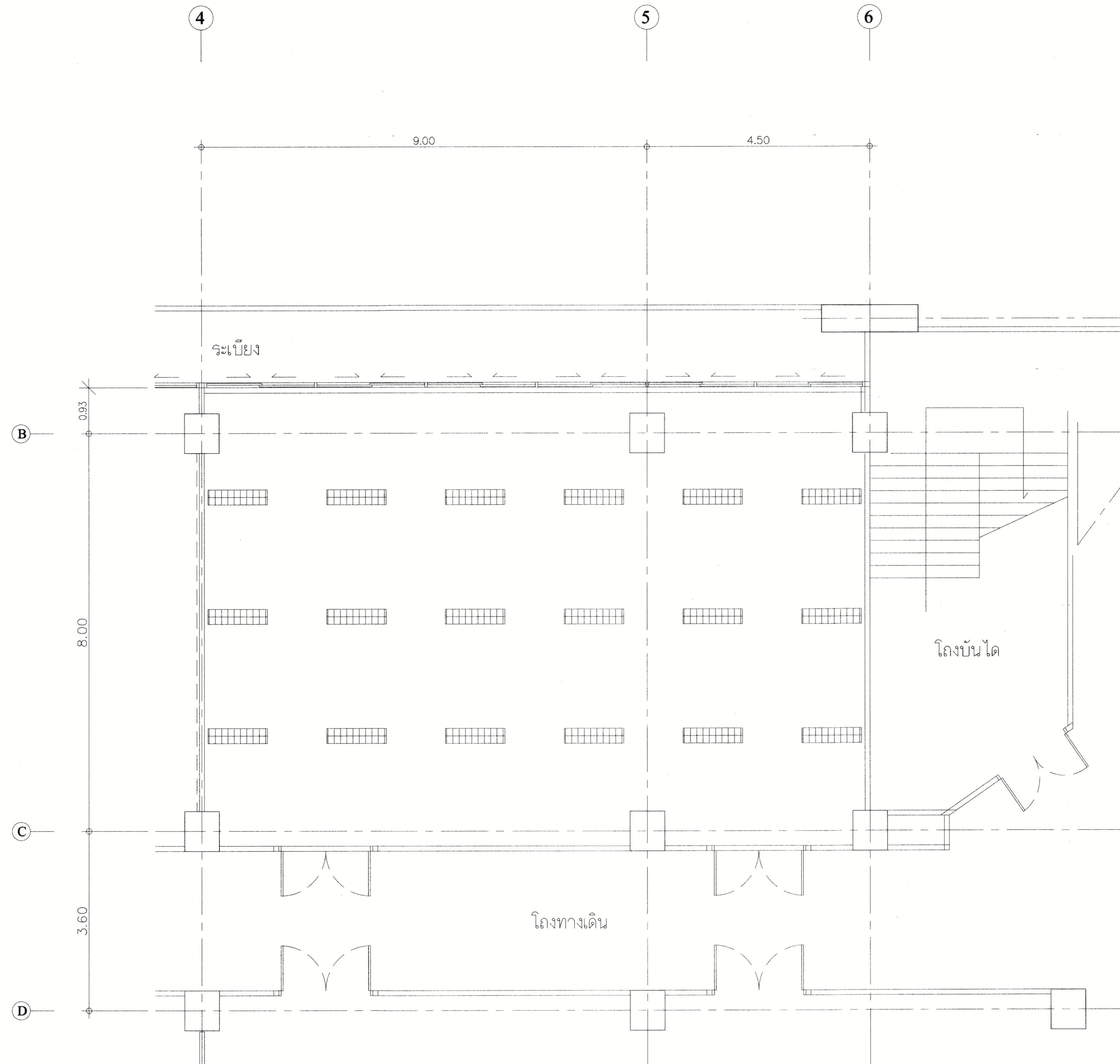
แปลน ไฟฟ้าแสงสว่าง ห้อง 806 , 808 ชั้น 8 (ก่อนปรับปรุง)
