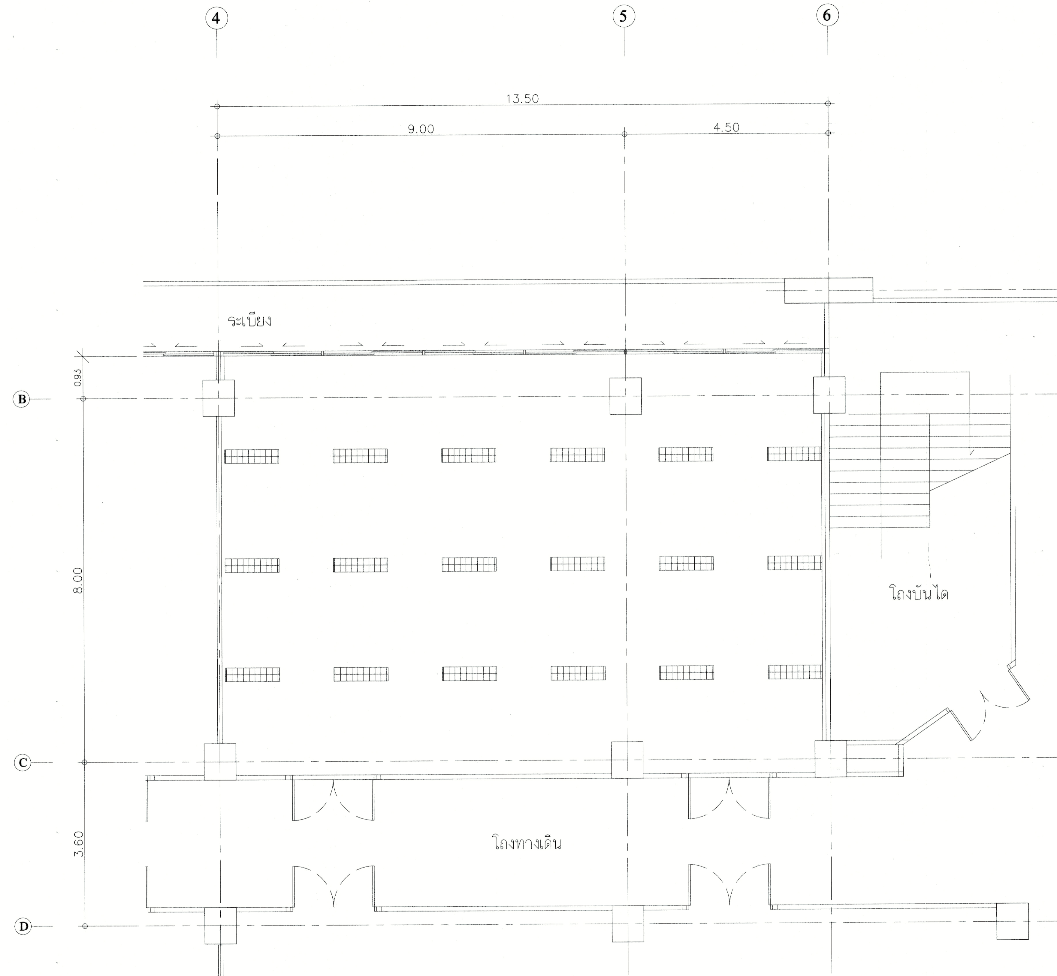
แปลน ไฟฟ้าแสงสว่าง ห้อง 606 , 608 ชั้น 6 (ก่อนปรับปรุง)
