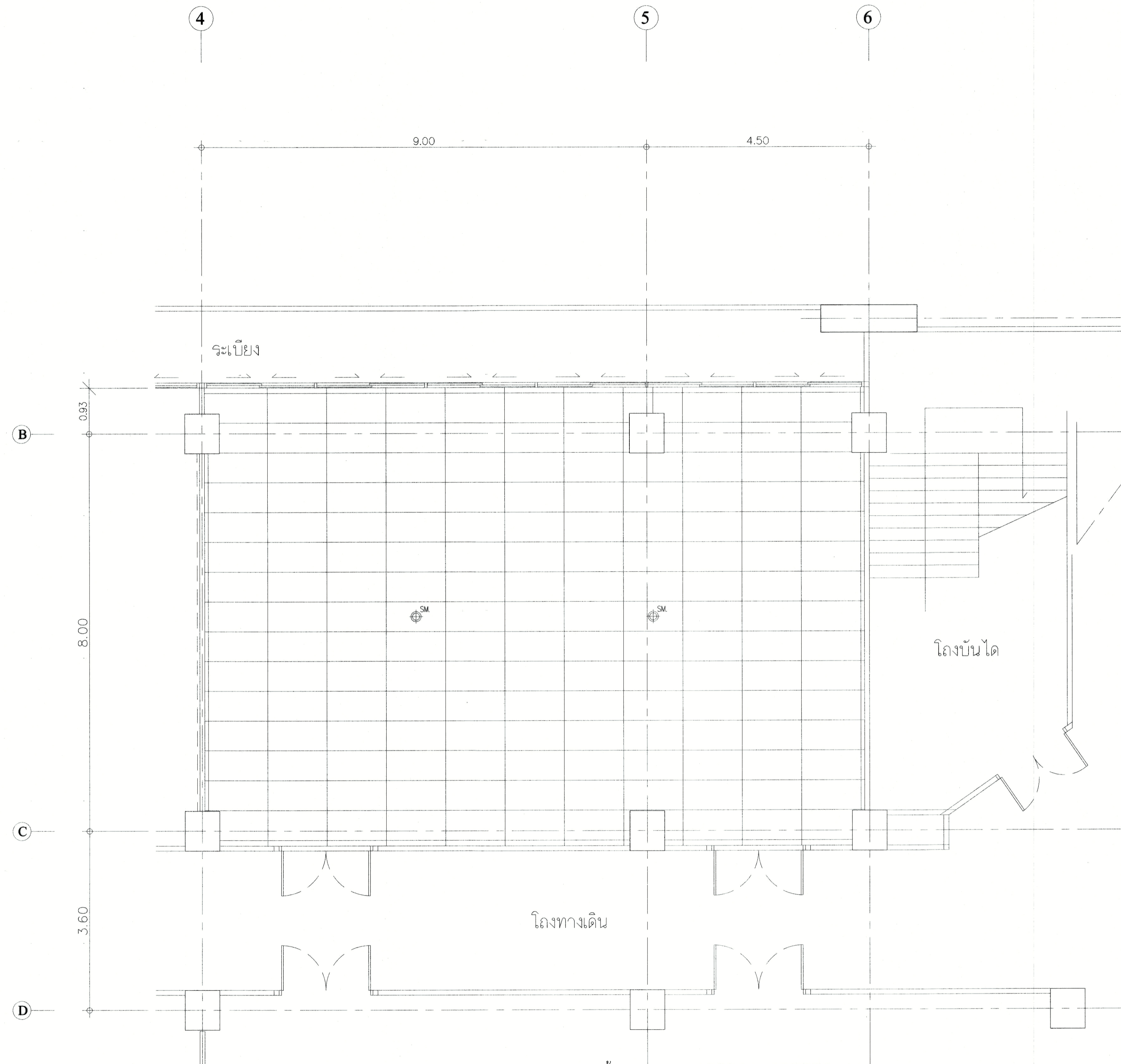
แปลน ตัวตรวจจับควันและความร้อน ห้อง 806 , 808 ชั้น 8 (ก่อนปรับปรุง)
