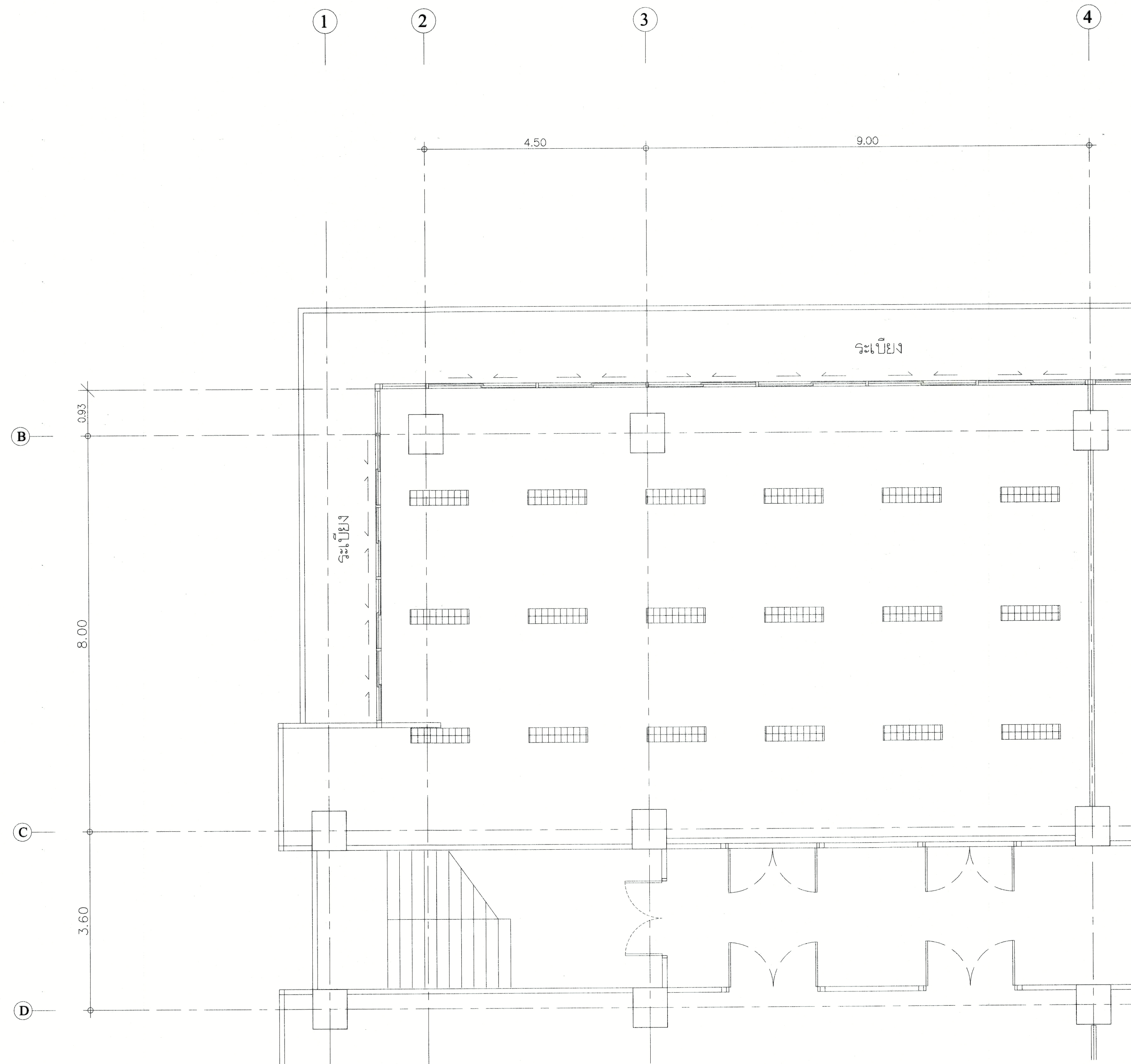
แปลน ไฟฟ้าแสงสว่าง ห้อง 802 , 804 ชั้น 8 (ก่อนปรับปรุง)
