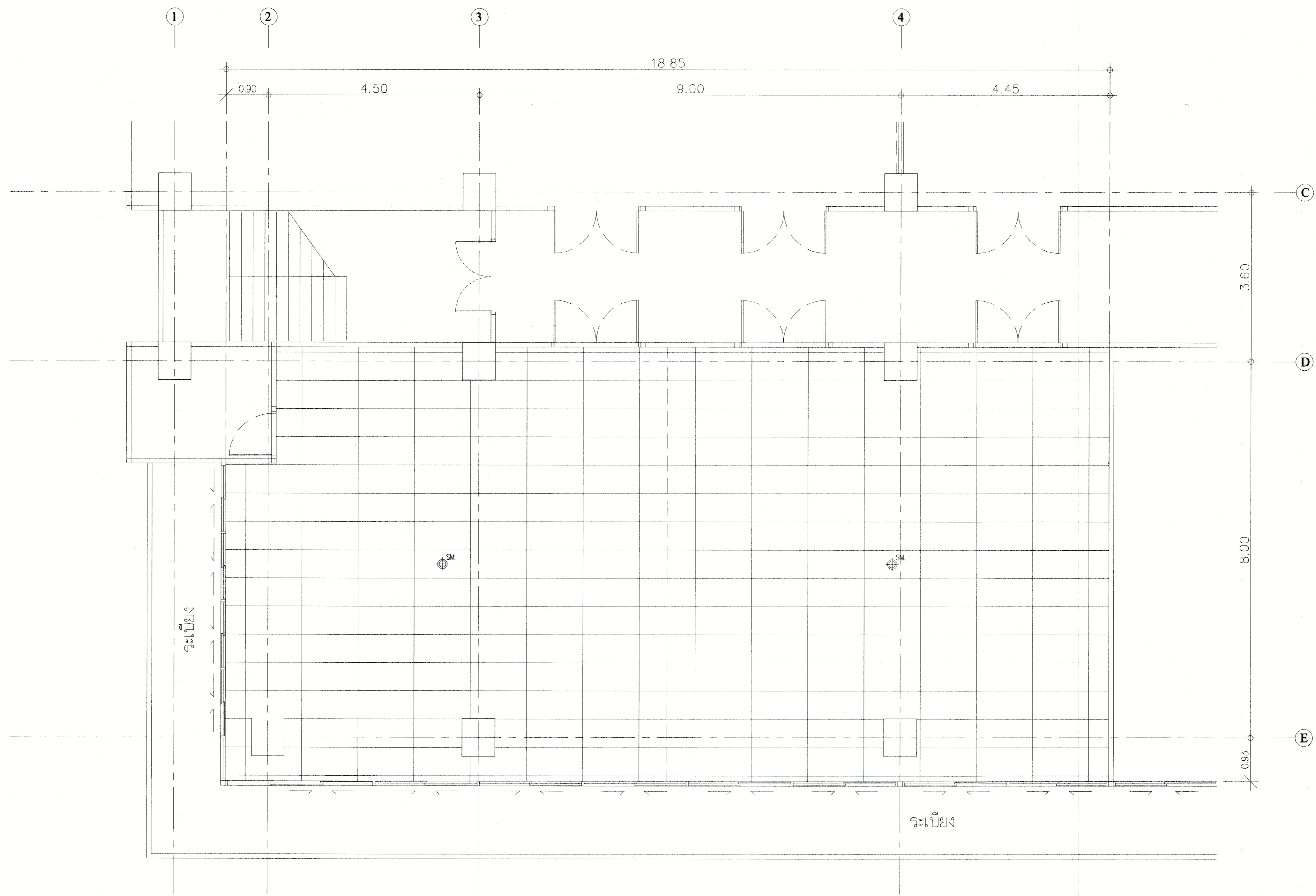
แปลน ตัวตรวจจับควันและความร้อน ห้อง 501 ชั้น 5 (ก่อนปรับปรุง)
