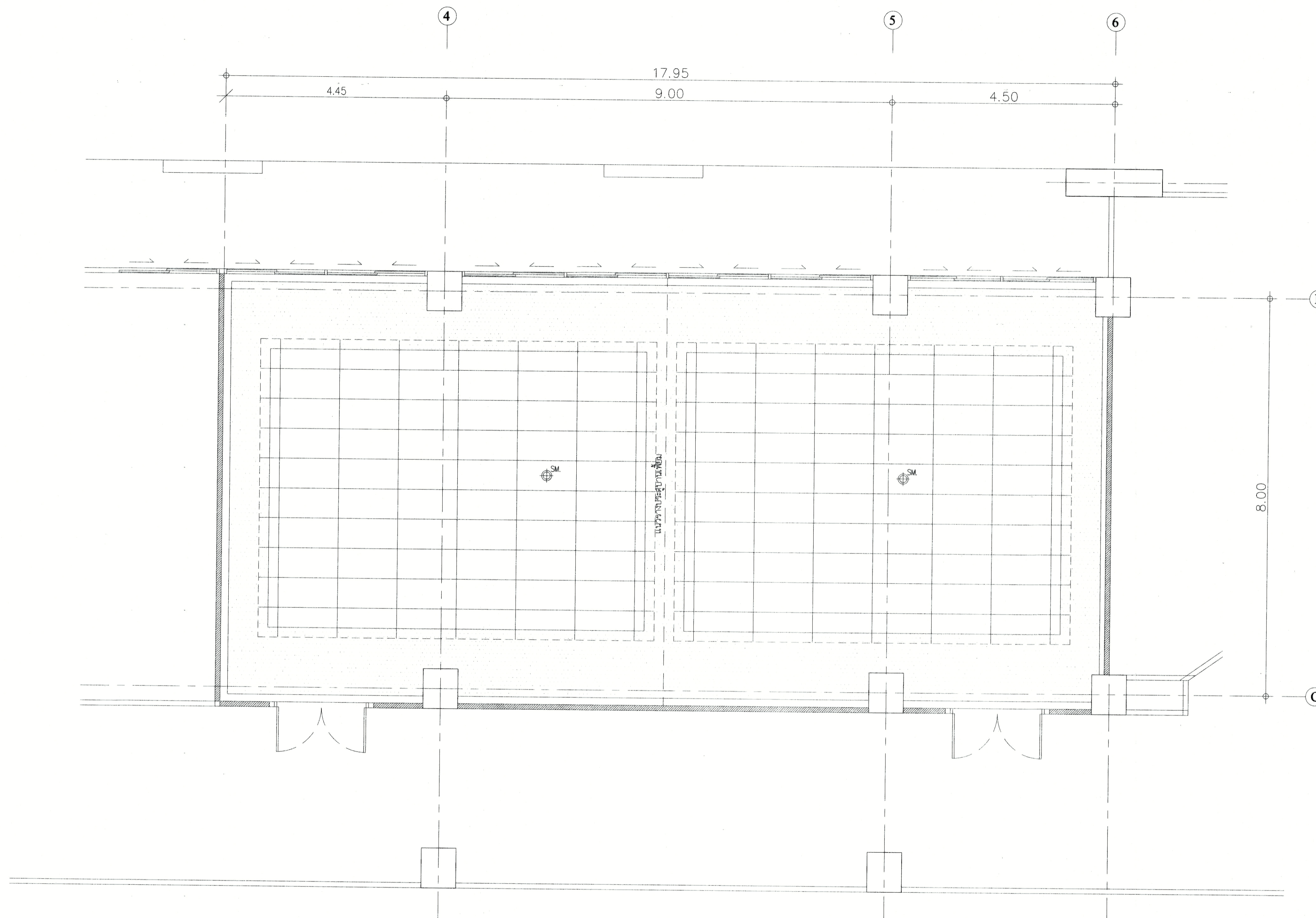
แปลน ตัวตรวจจذبคลื่นและความร้อน สำนักงาน ชั้น 2 (ก่อนปรับปรุง)
