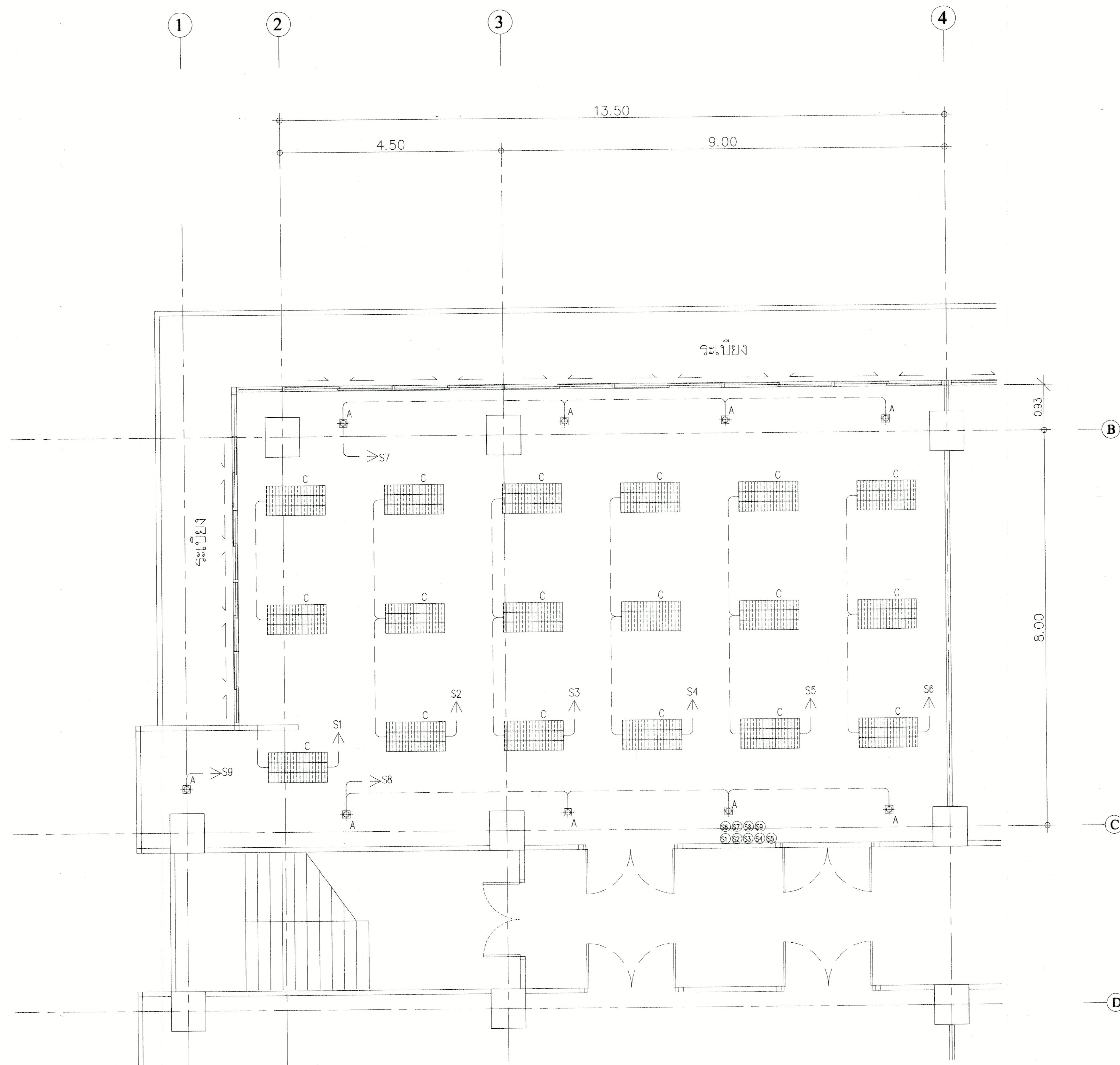
แปลน ไฟฟ้าแสงสว่าง ห้อง 802 , 804 ชั้น 8 (หลังปรับปรุง) ระบบไฟต่อกับตู้คอนโทรลเดิม ให้พร้อมใช้งาน
