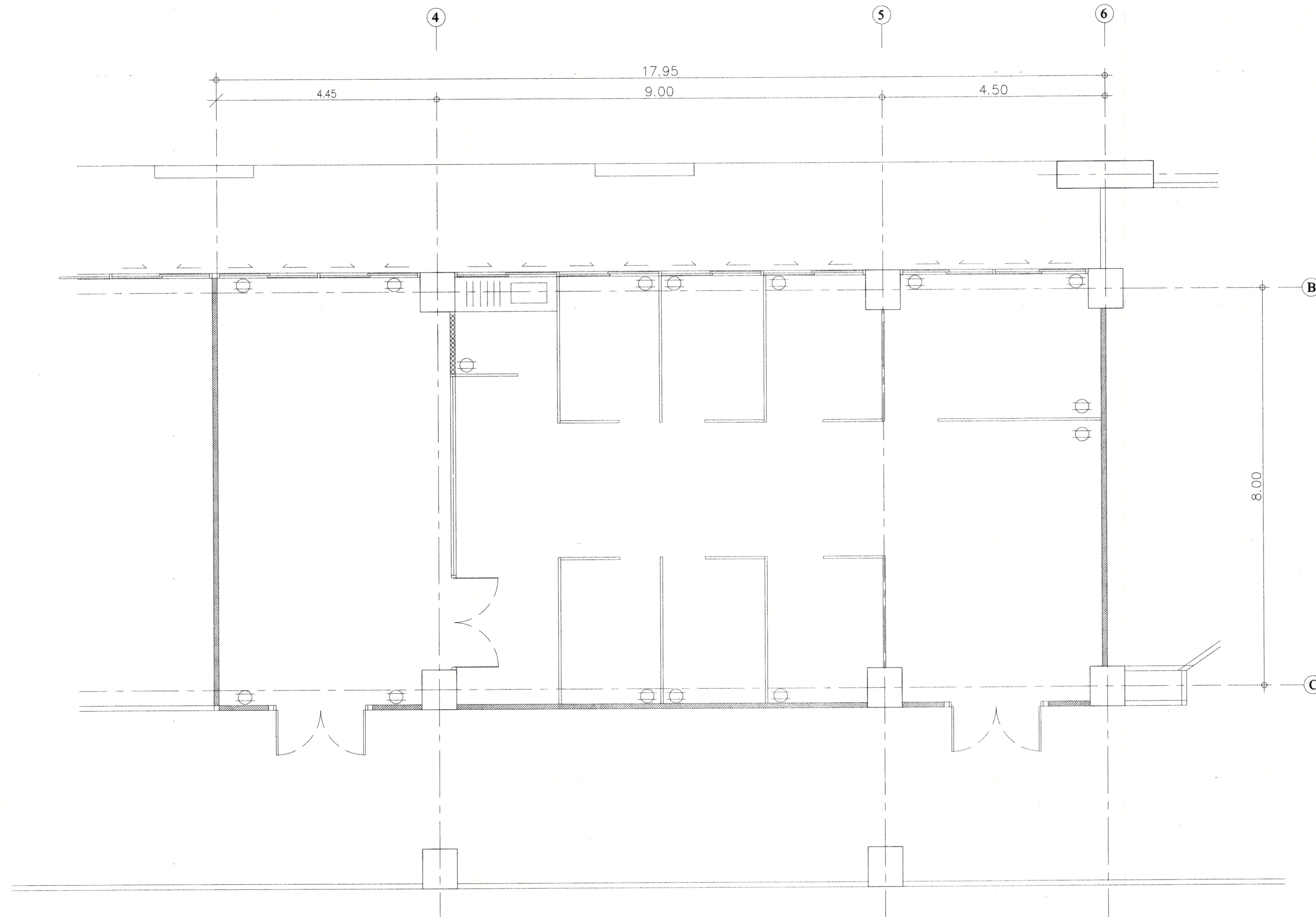
แปลน เค้าเสียบ สำนักงาน ชั้น 2 (ไม่รวม) 150 (หลังปรับปรุง) ระบบไฟฟ้ากับตู้คอนโทรลเดิม ให้พร้อมใช้งาน
