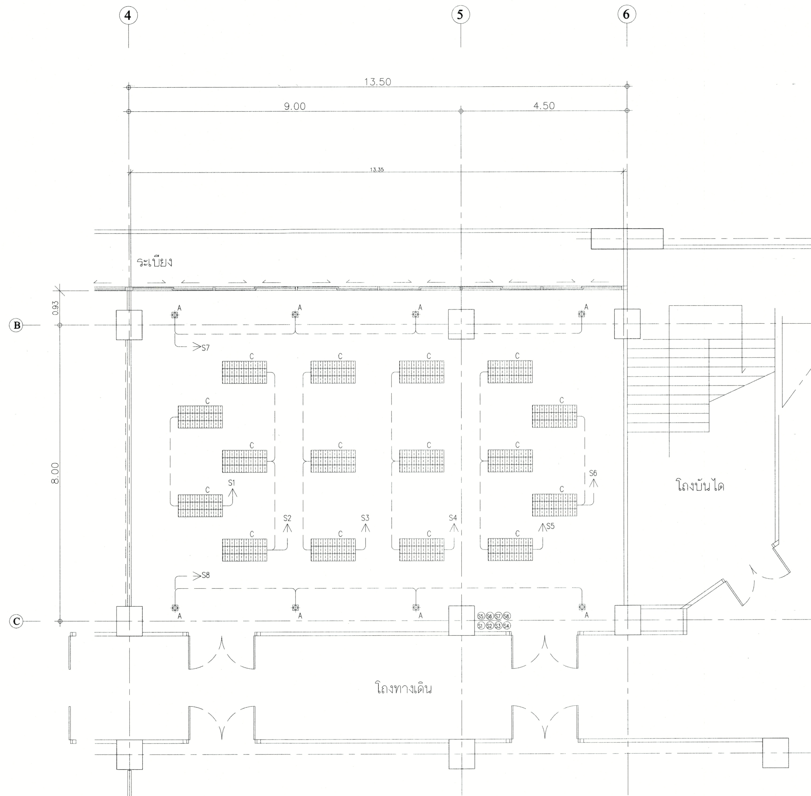
150 แบนไฟฟ้าแสงสว่าง ห้อง 806, 808 ชั้น 8 (หลังปรับปรุง) ระบบไฟติดกับตู้คอนโทรลเดิม ให้พร้อมใช้งาน
