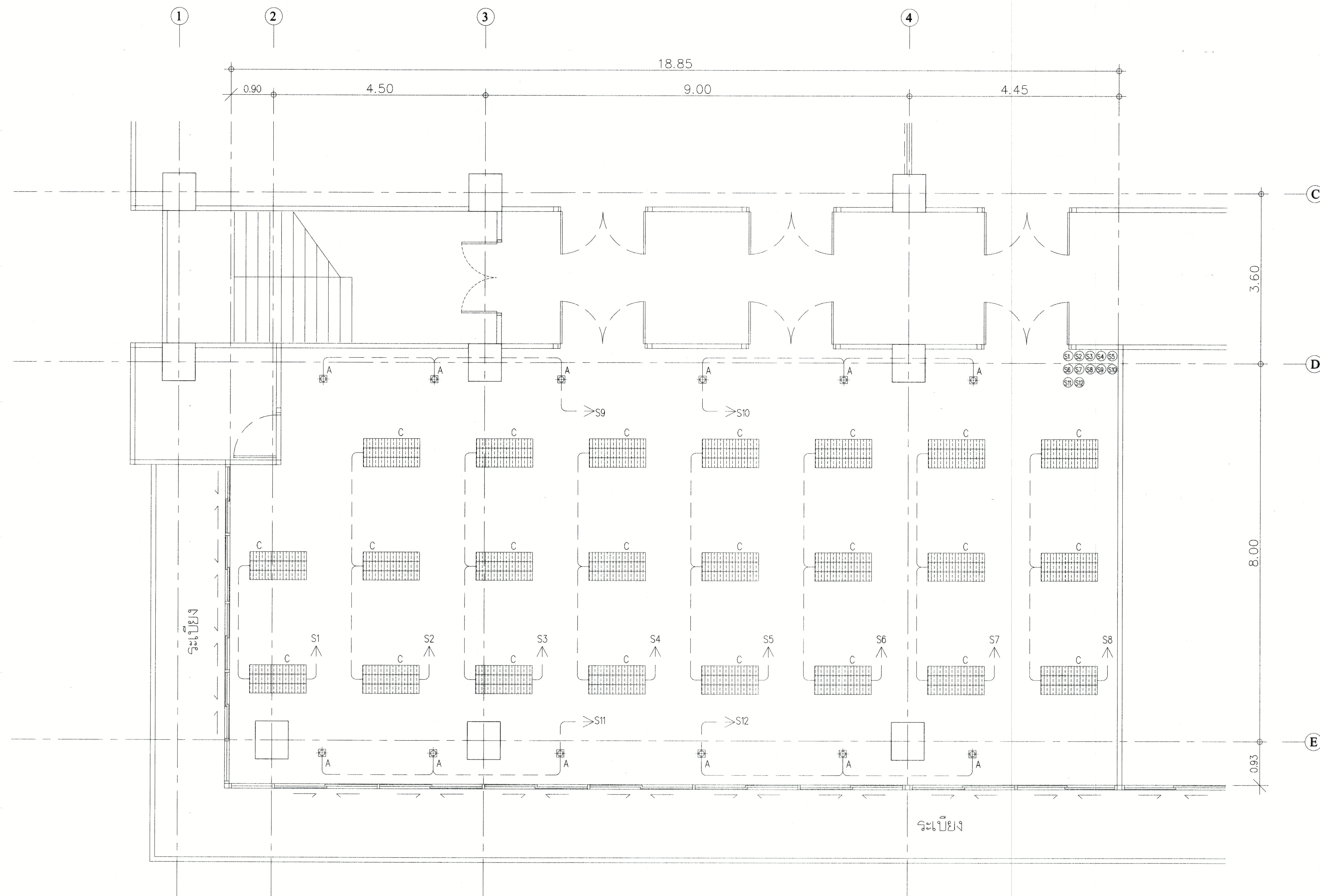
150 แปลน ไฟฟ้าแสงสว่าง ห้อง 501 ชั้น 5 (หลังปรับปรุง) ระบบไฟต่อกับตู้คอนโทรลเดิม ให้พร้อมใช้งาน
