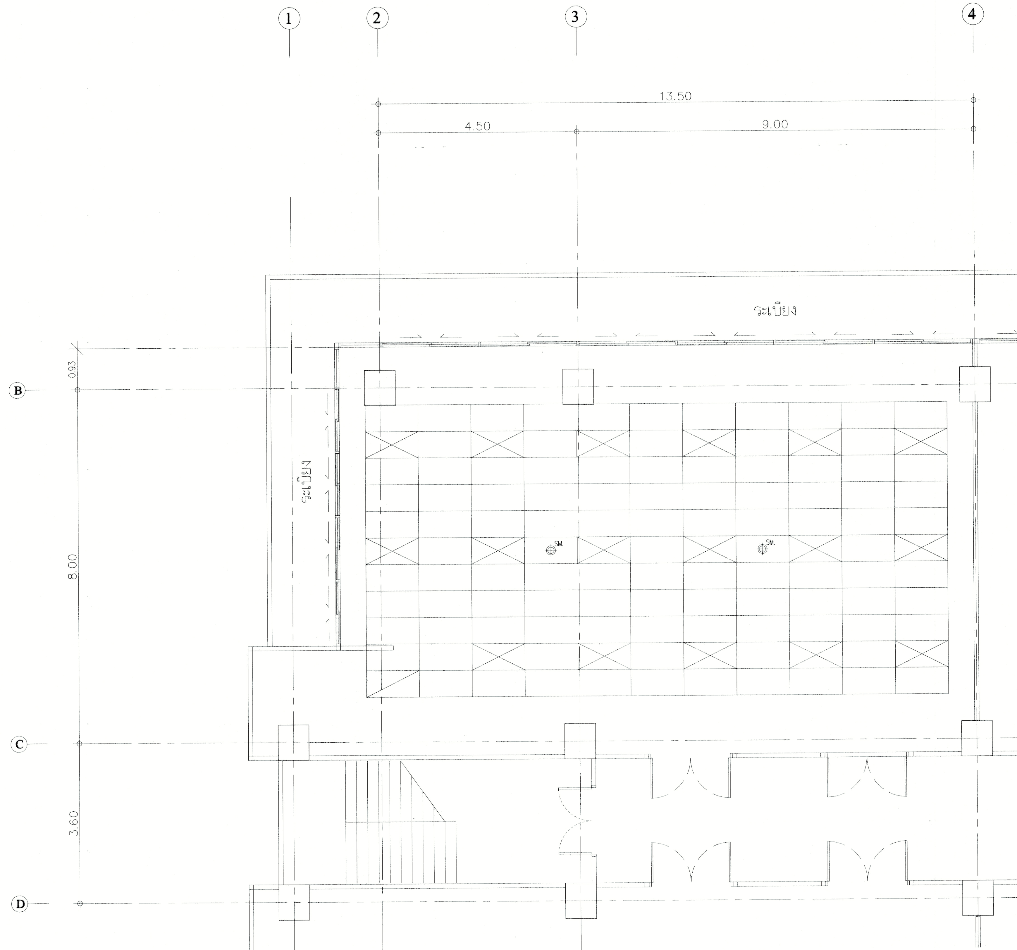
แบบแปลน ตัวตรวจจับควันและความร้อน ห้อง 802 , 804 ชั้น 8 (หลังปรับปรุง)
