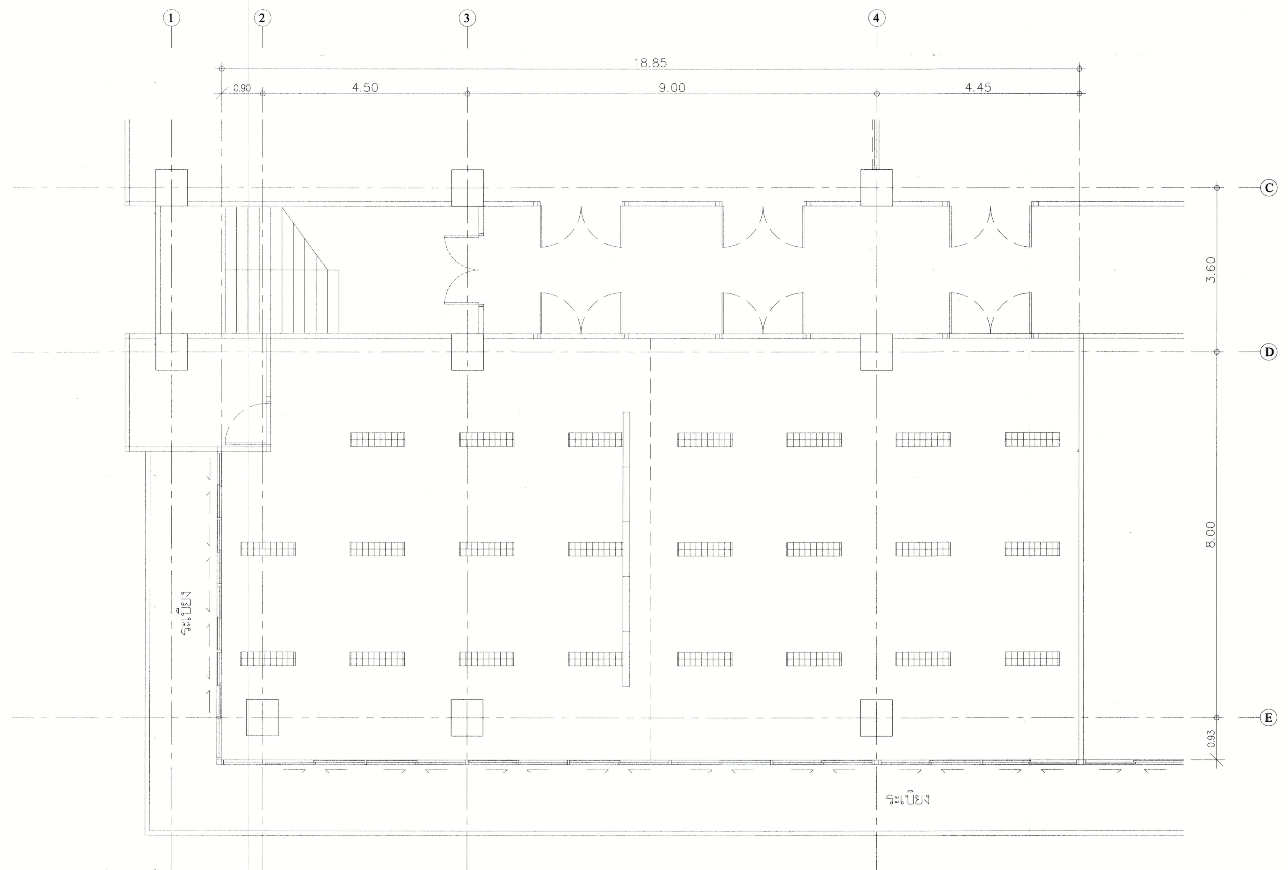
แปลน ไฟฟ้าแสงสว่าง ห้อง 501 ชั้น 5 150 (ก่อนปรับปรุง)
