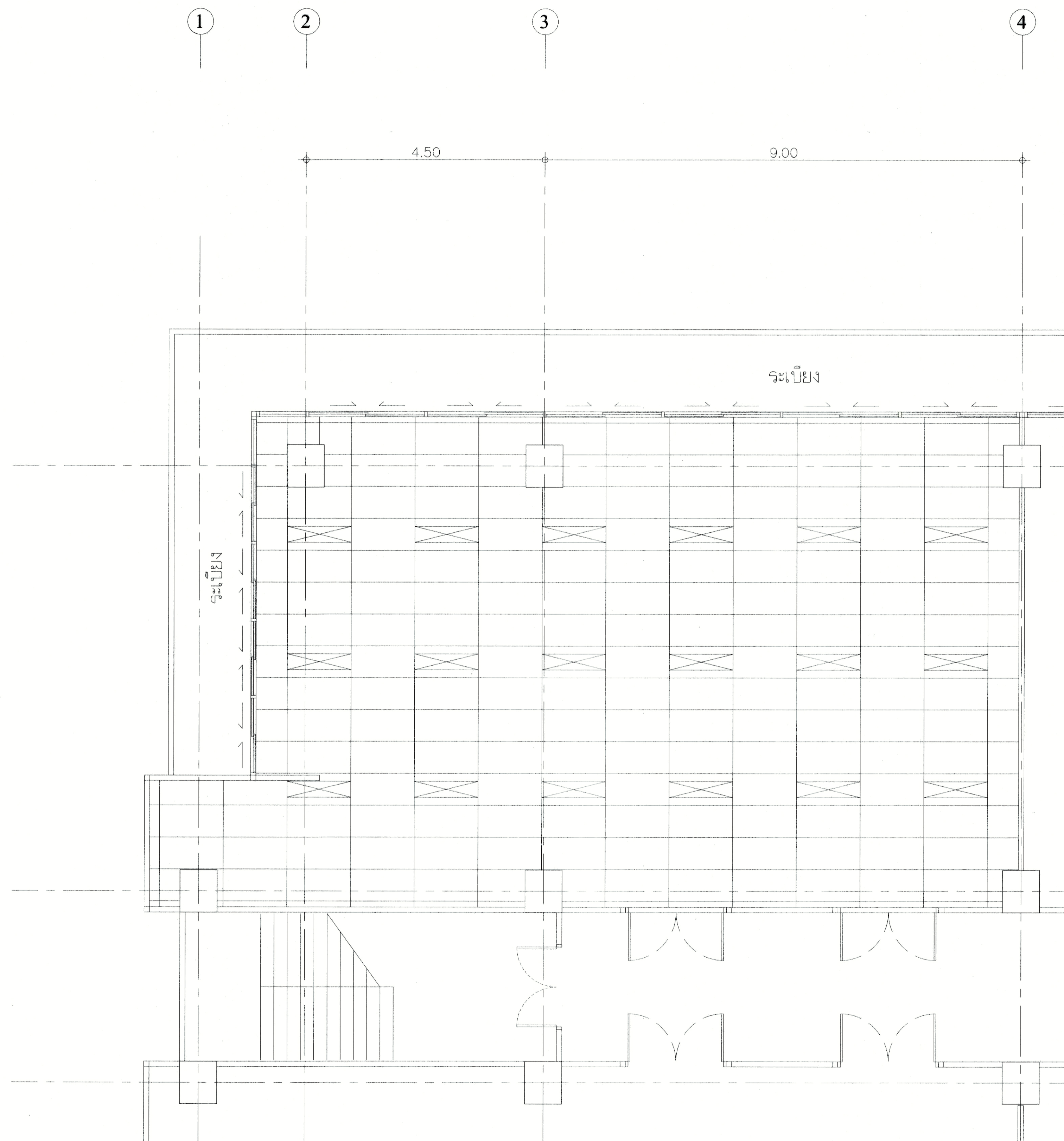
แปลน ฝ้าเพดาน ห้อง 802 , 804 ชั้น 8 (ก่อนปรับปรุง)
