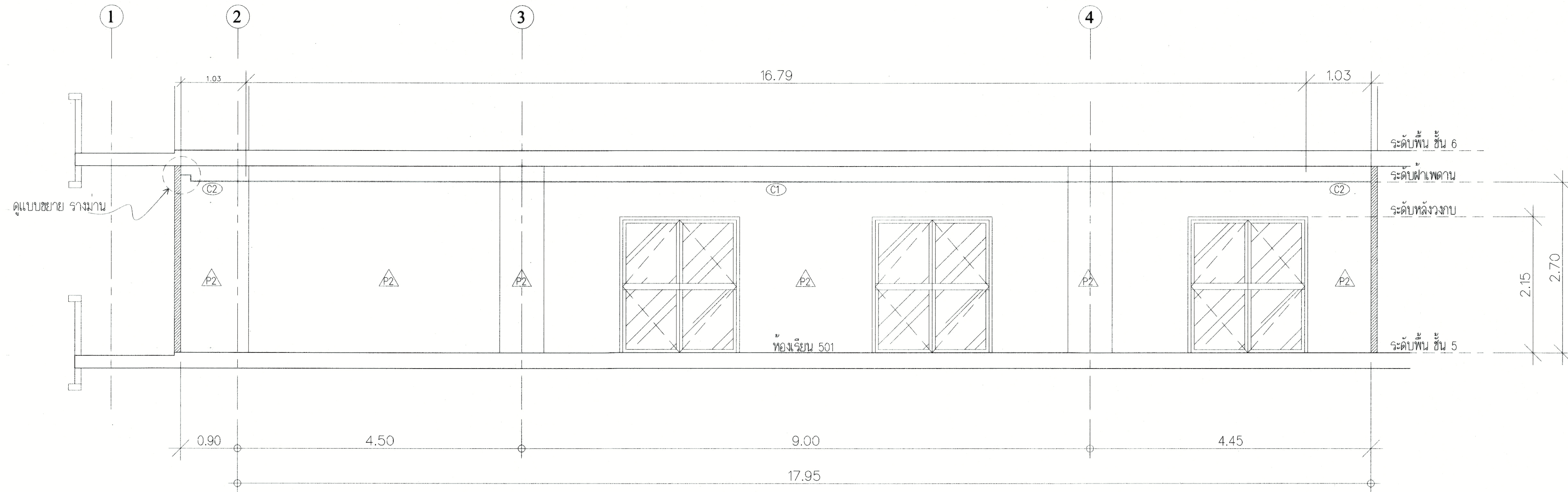
รูปตัด A 1:40 (หลังปรับปรุง)
