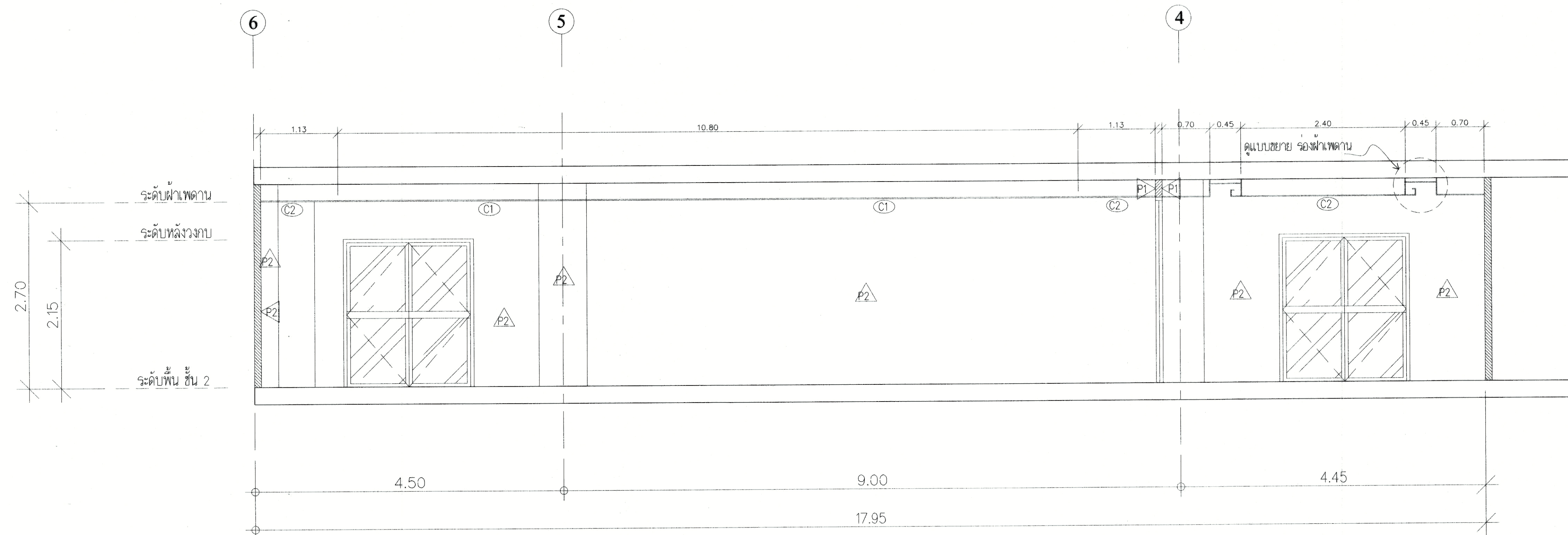
รูปตัด D 1:40 (หลังปรับปรุง)
