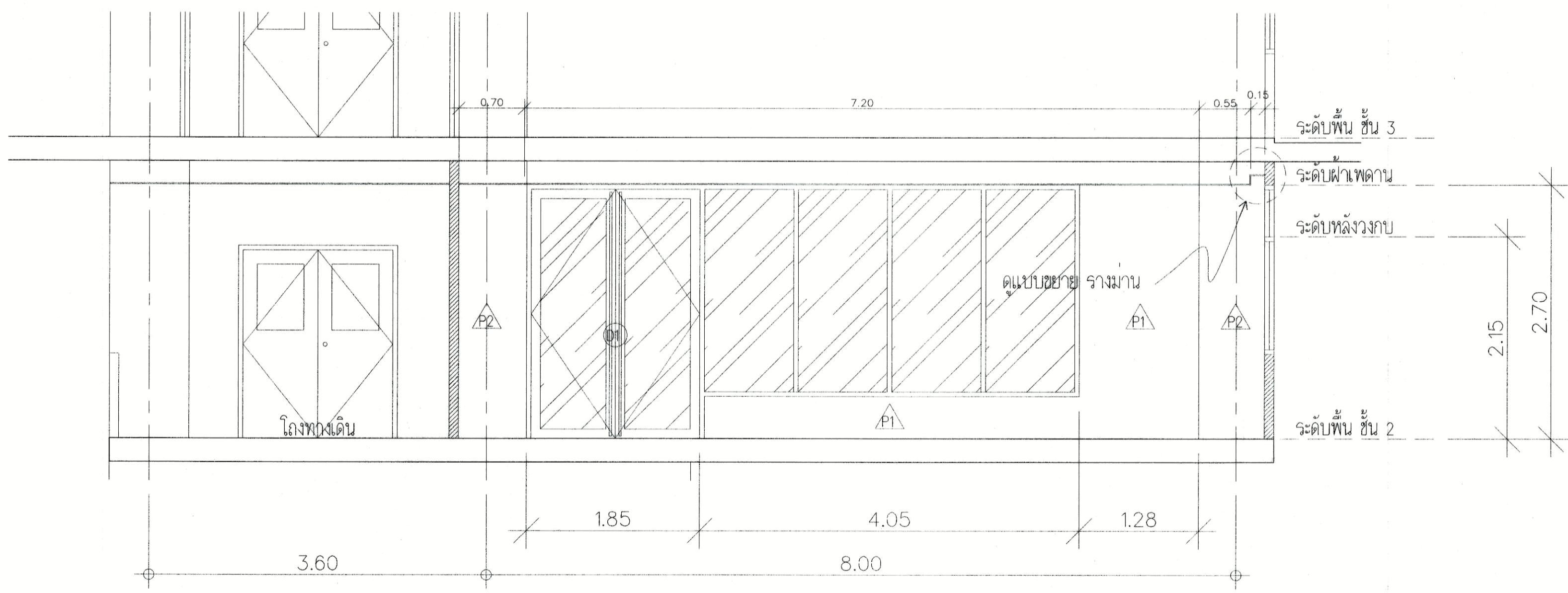
รูปตัด B 1:40 (หลังปรับปรุง)
