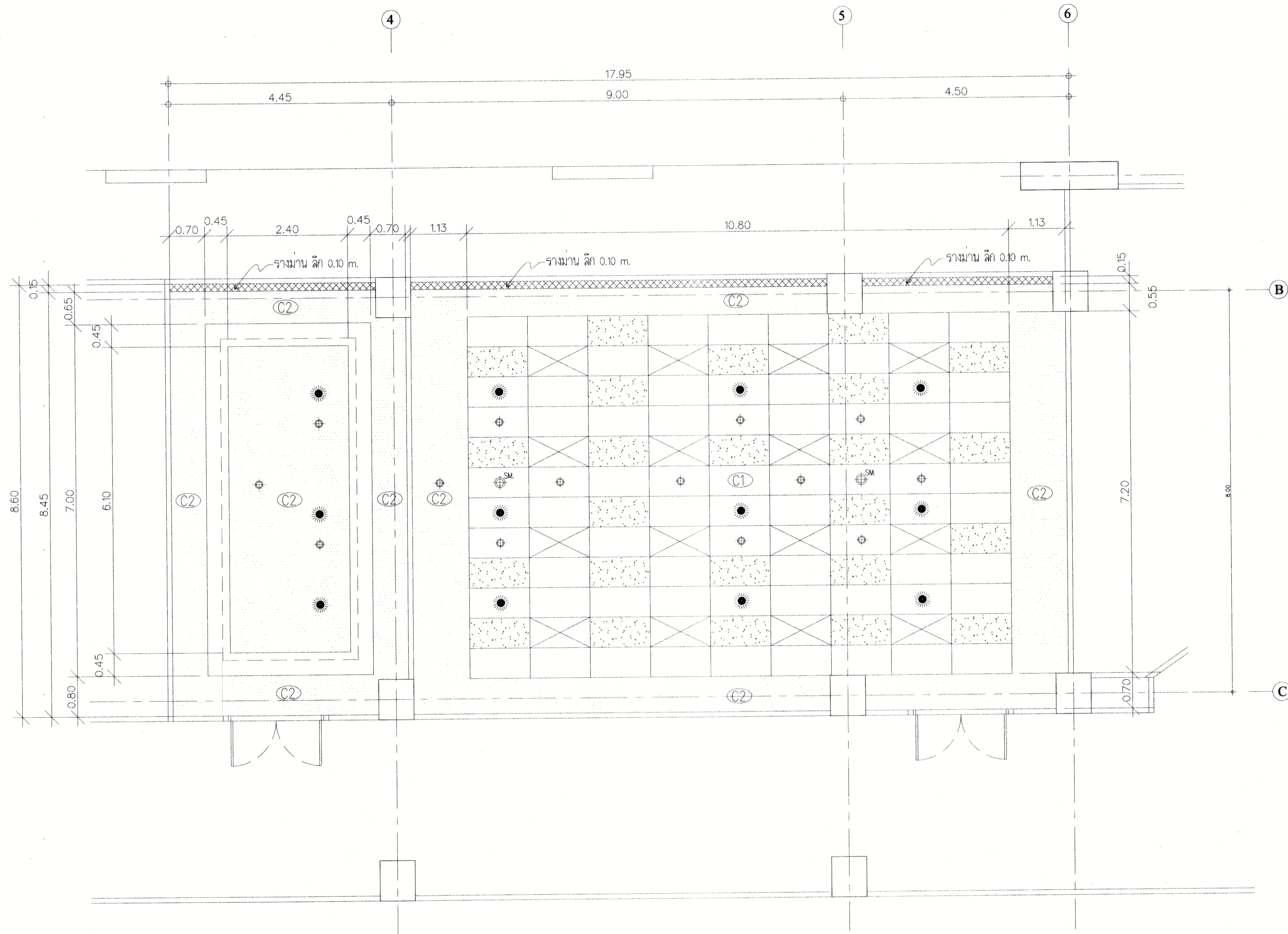
แปลน ฝ้าเพดาน สำนักงาน ชั้น 2 150 (หลังปรับปรุง)
