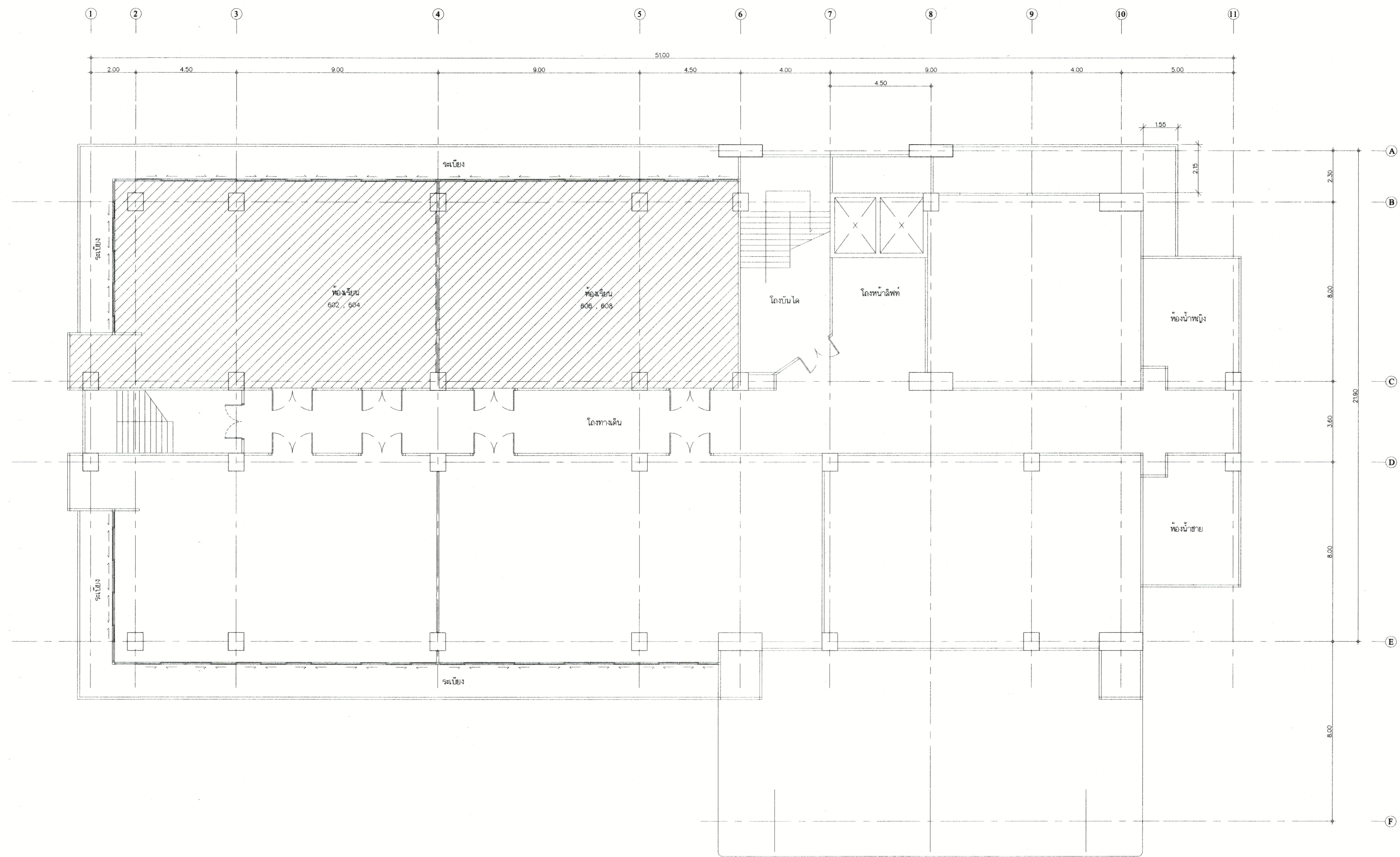
แปลน ชั้น 6 175 (หลังปรับปรุง)
