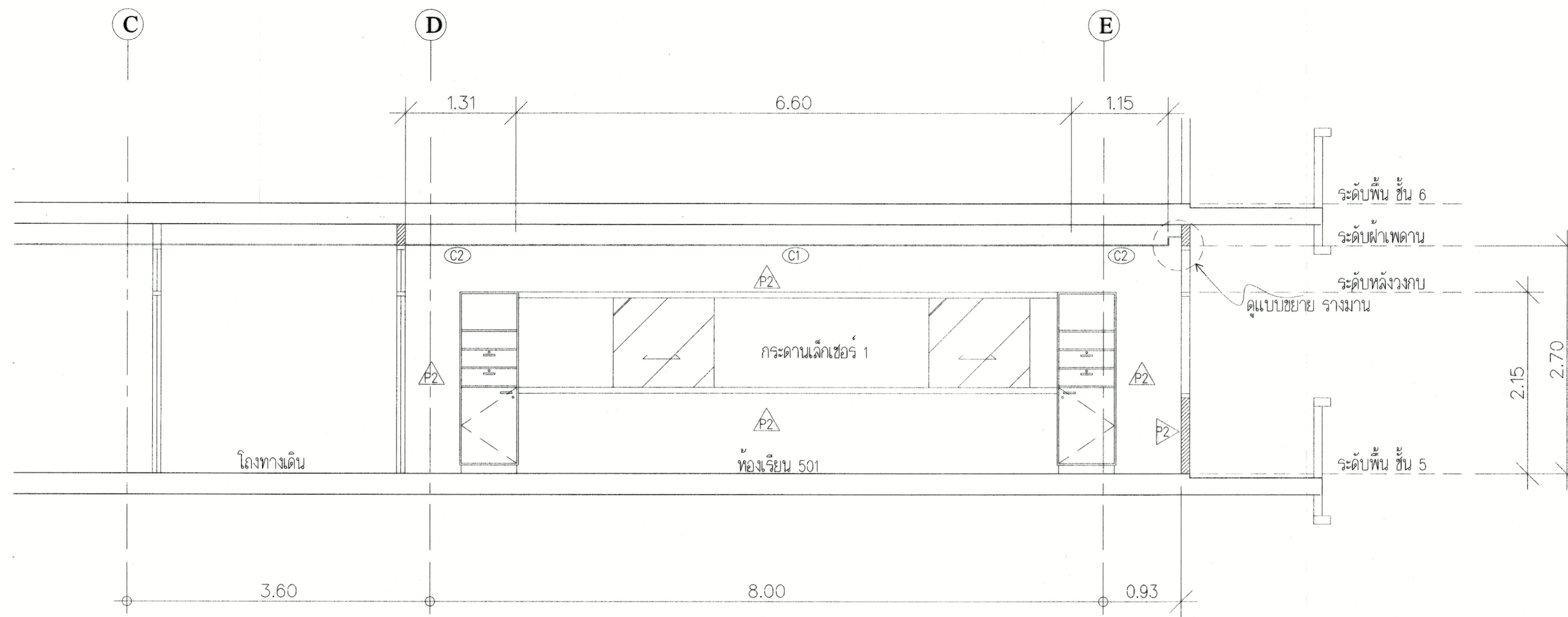
รูปตัด C 1:40 (หลังปรับปรุง)
