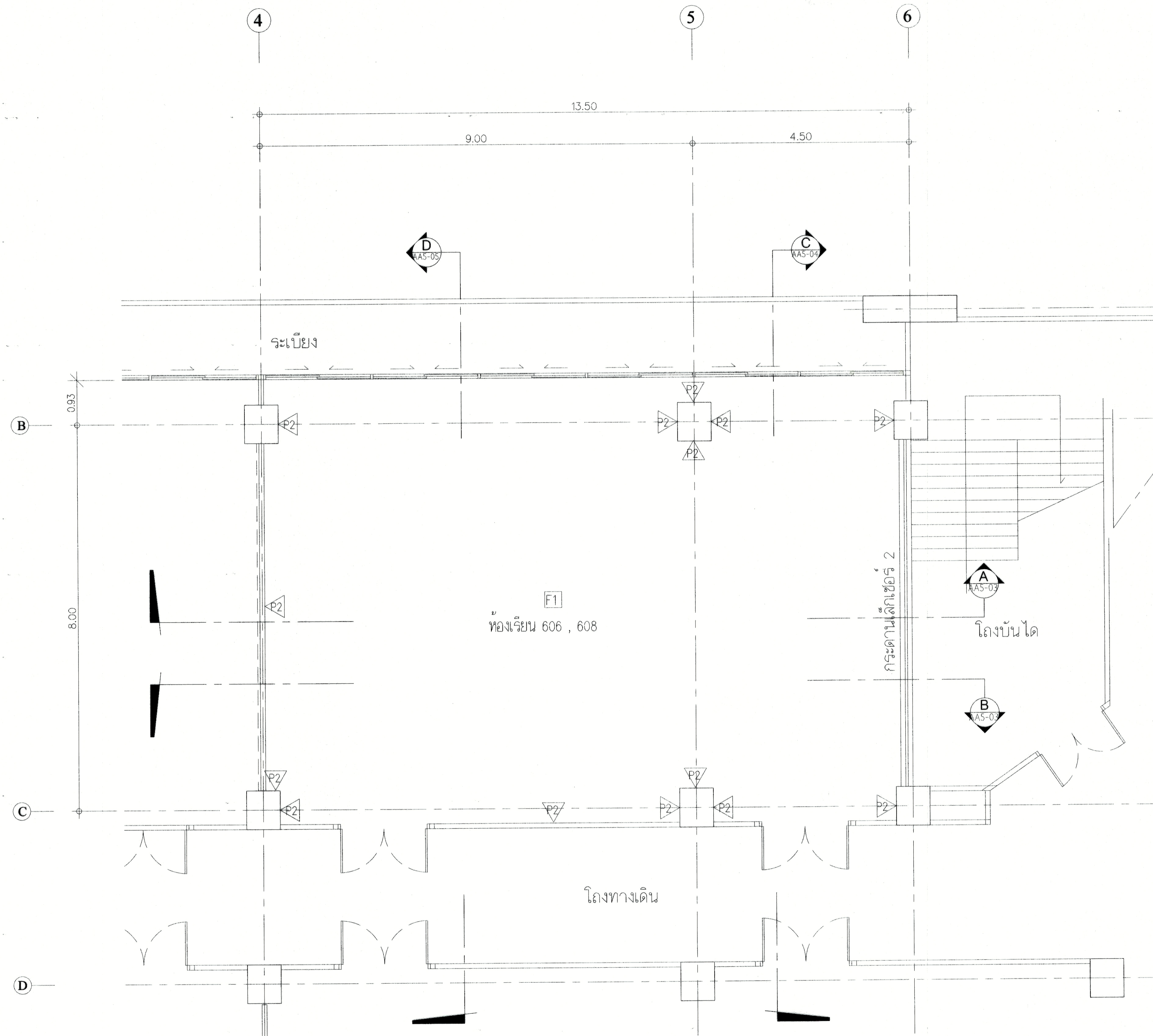
แปลน ขยายห้อง 606, 608 ชั้น 6 (หลังปรับปรุง)
