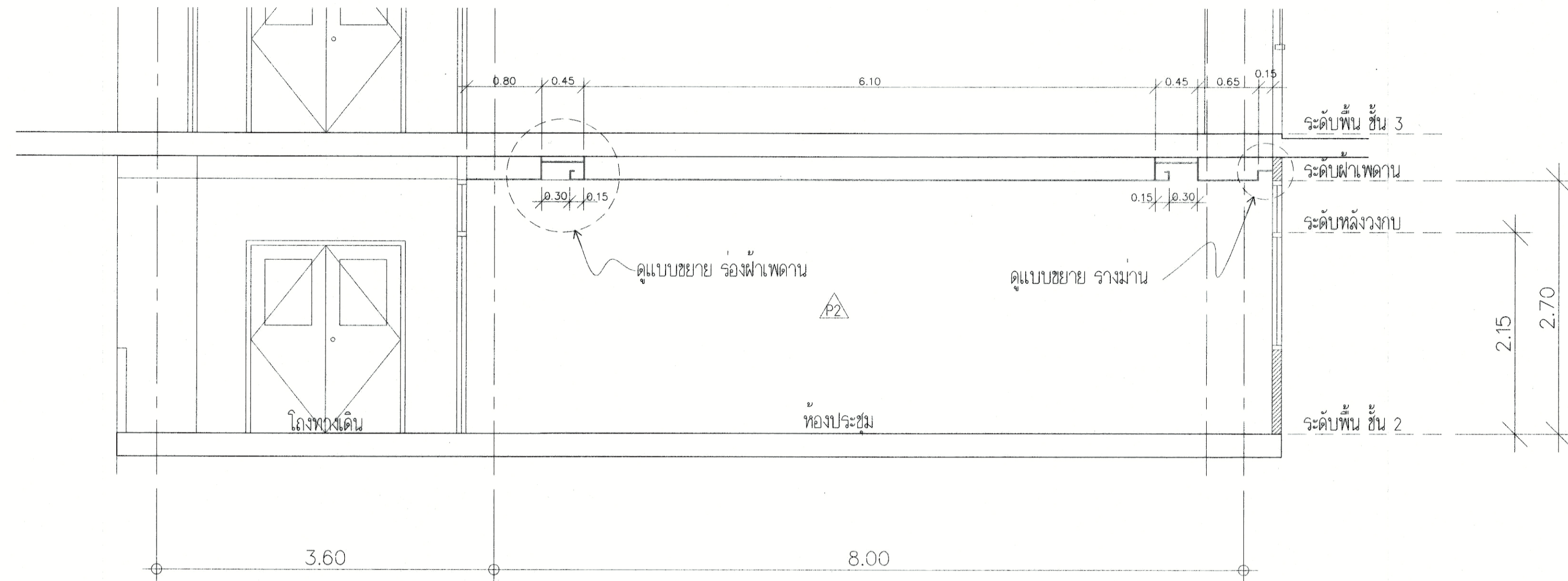
รูปตัด A 1:40 (หลังปรับปรุง)
