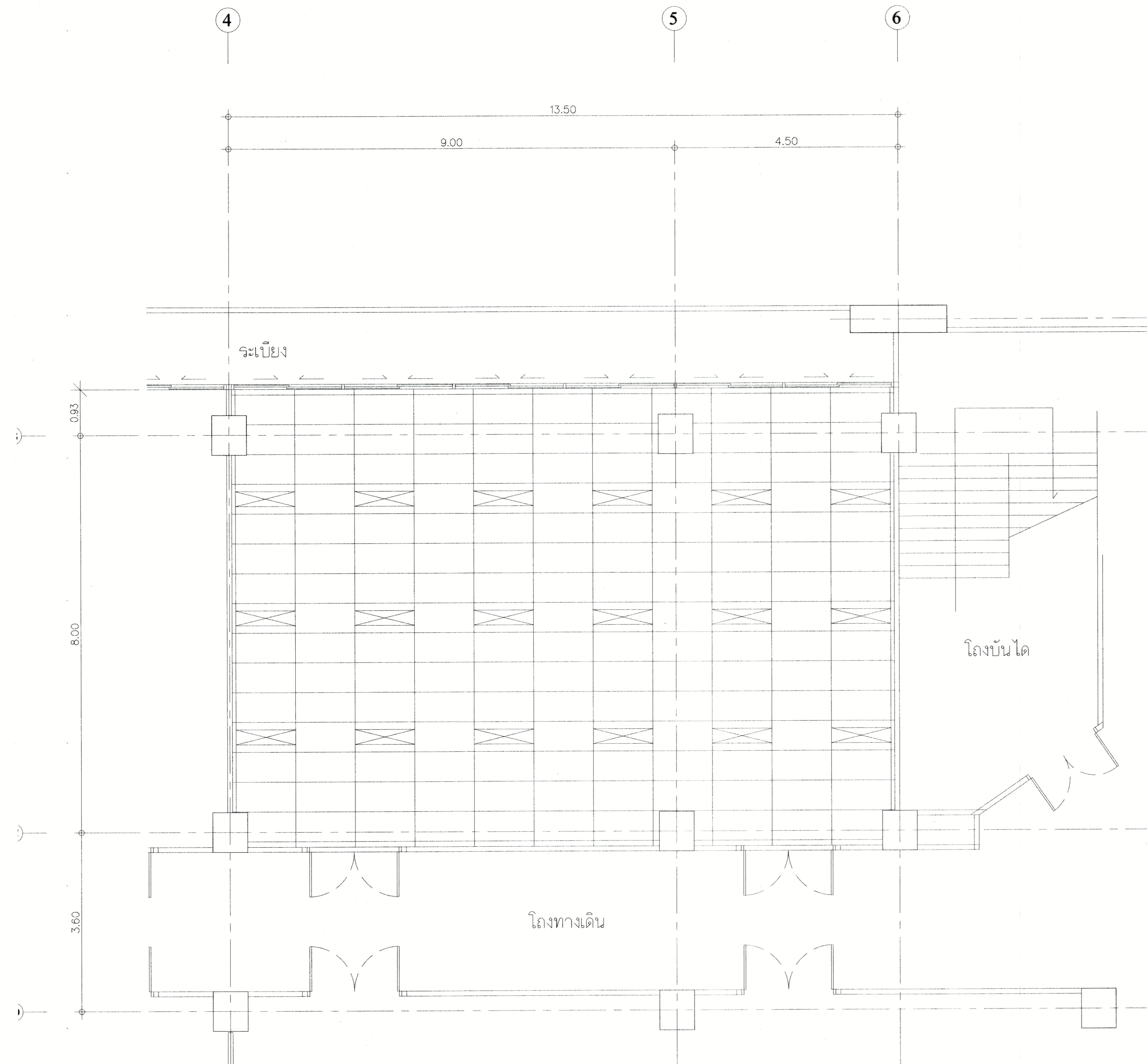
แปลน ฝ้าเพดาน ห้อง 806 , 808 ชั้น 8 (ก่อนปรับปรุง)
