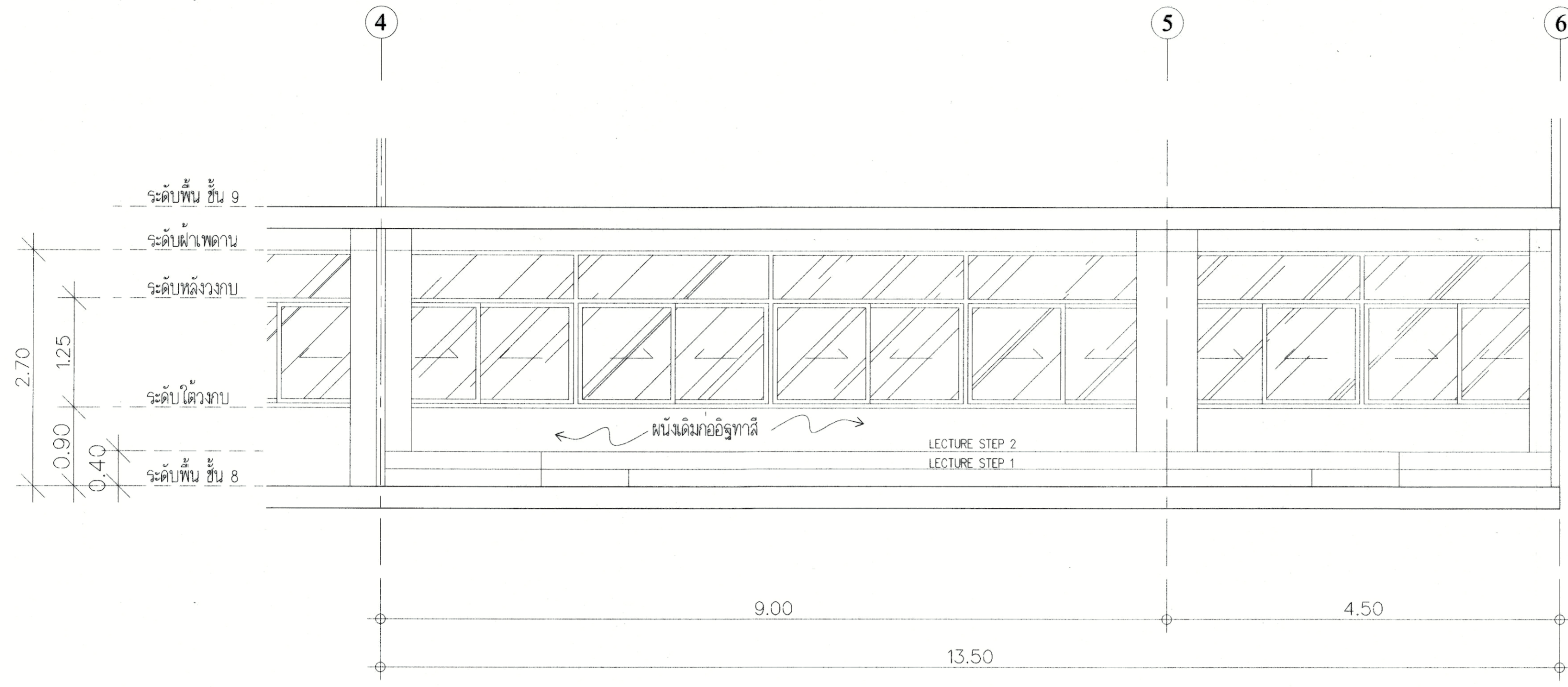
รูปตัด A 1:40 (ก่อนปรับปรุง)
