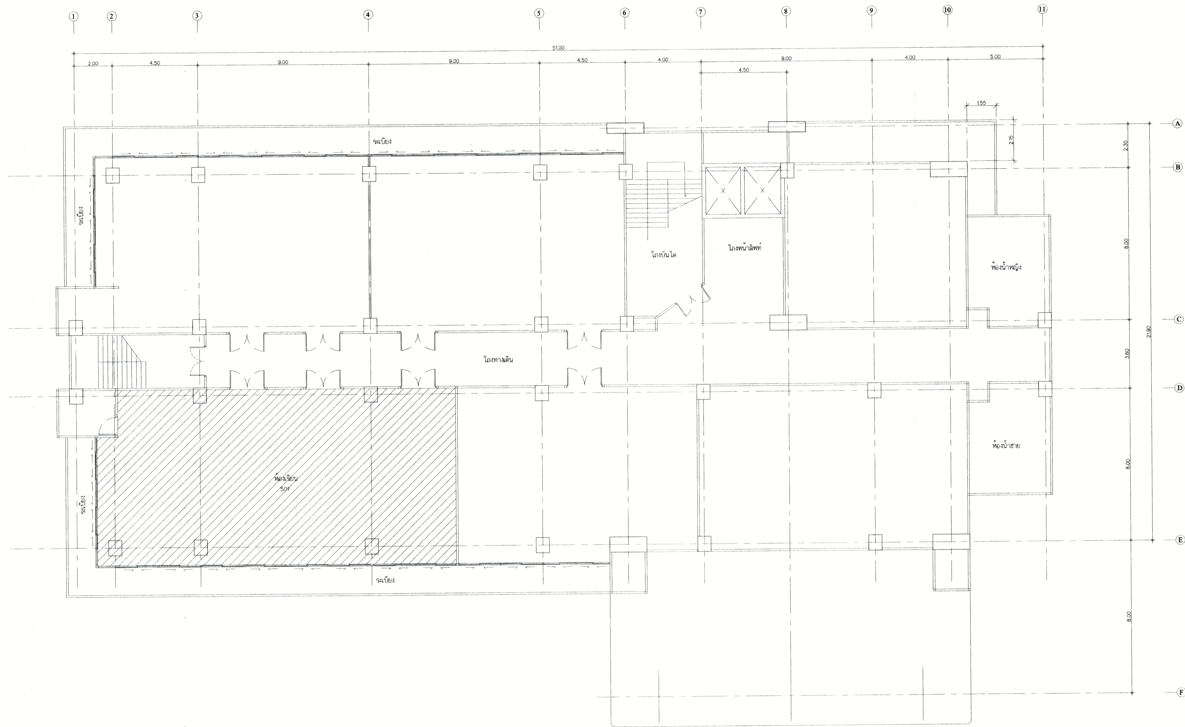
แปลน ชั้น 5 175 (หลังปรับปรุง)
