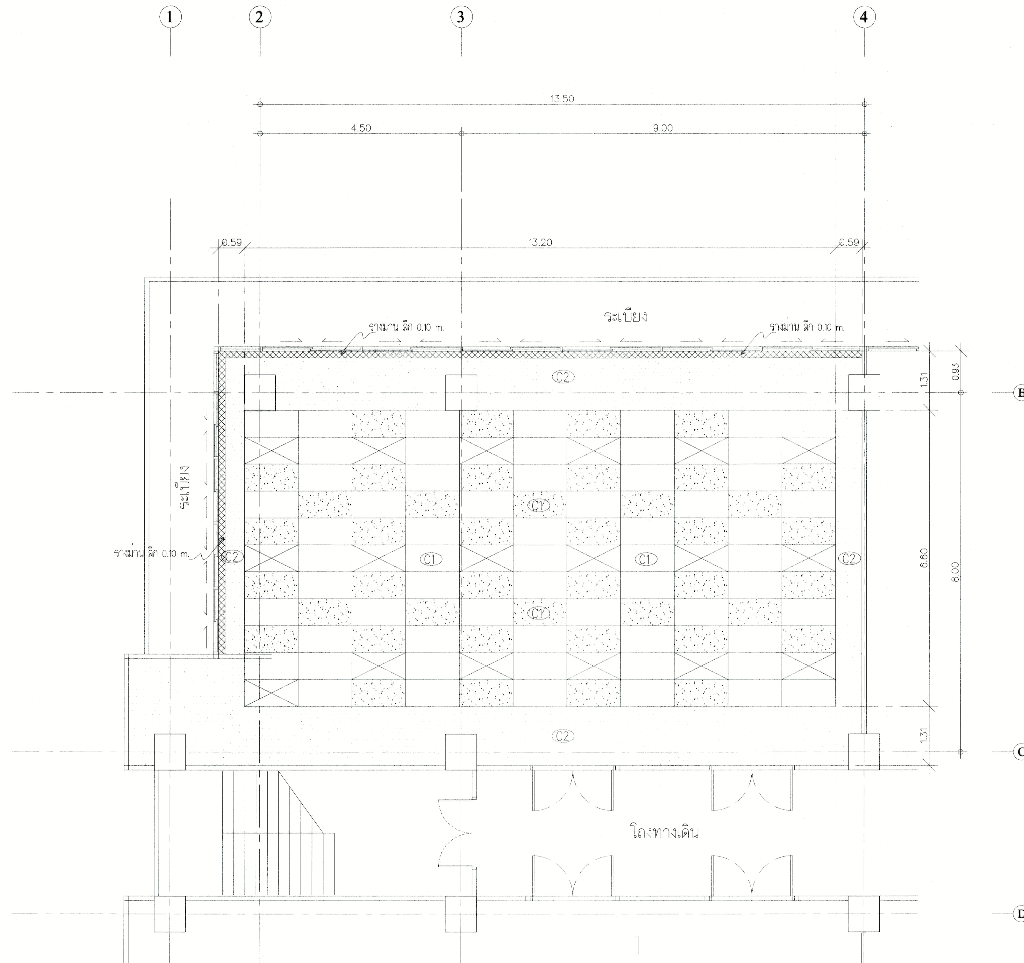
แปลน ฝ้าเพดาน ห้อง 602 , 604 ชั้น 6 (หลังปรับปรุง)
