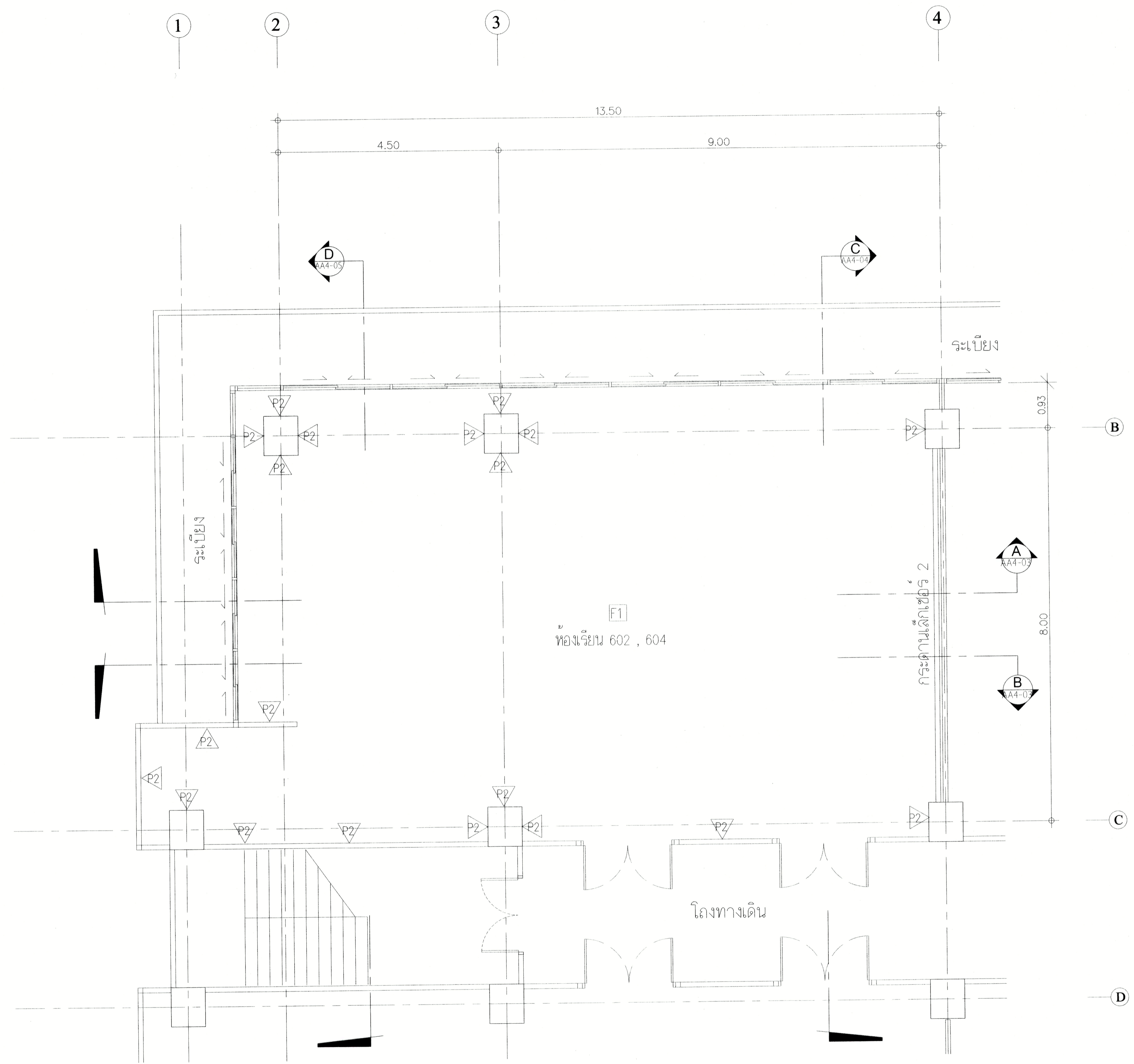
แปลน ขยายห้อง 602, 604 ชั้น 6 150 (หลังปรับปรุง)
