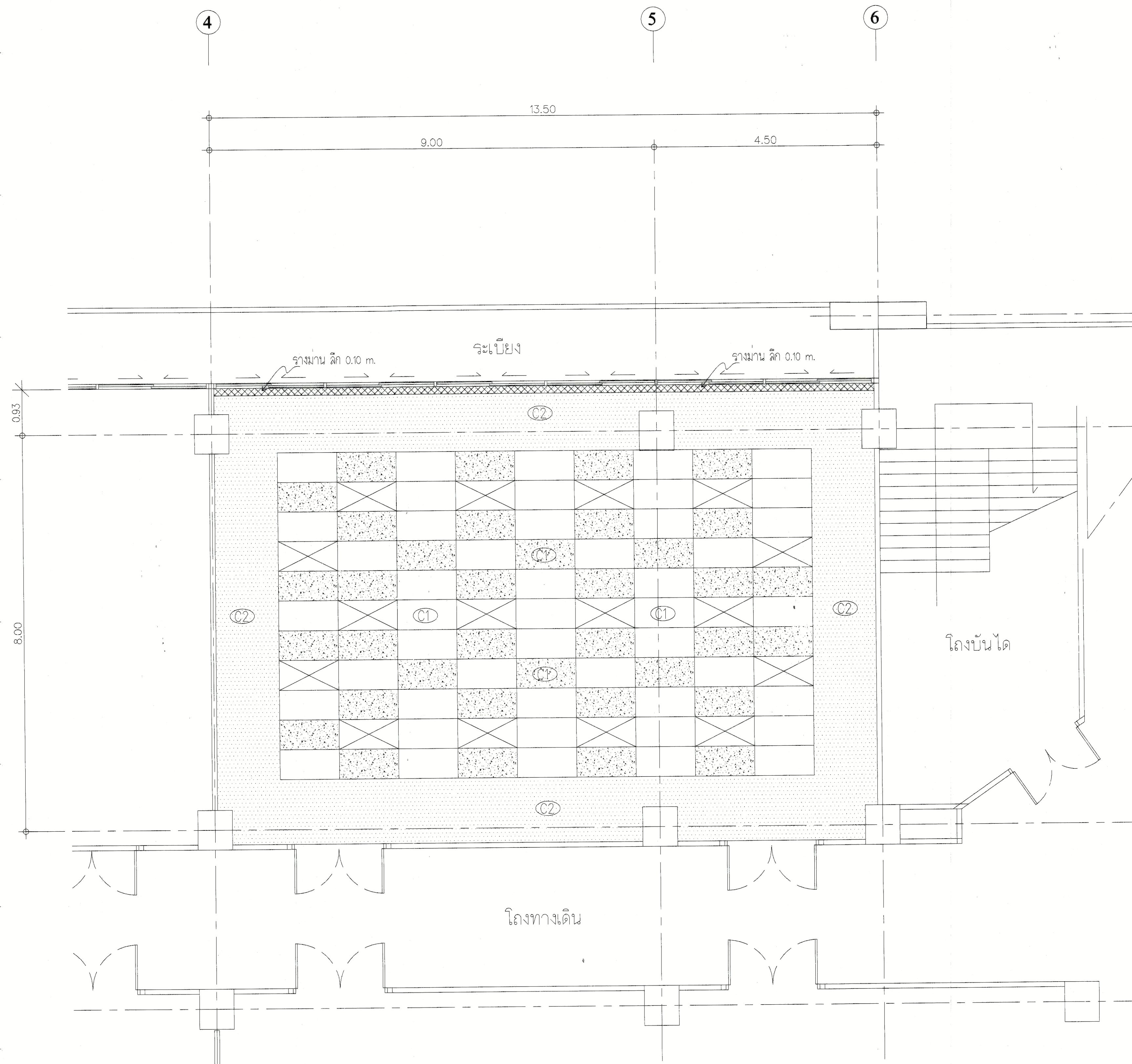
แปลน ฝ้าเพดาน ห้อง 606 , 608 ชั้น 6 (หลังปรับปรุง) 1:50
