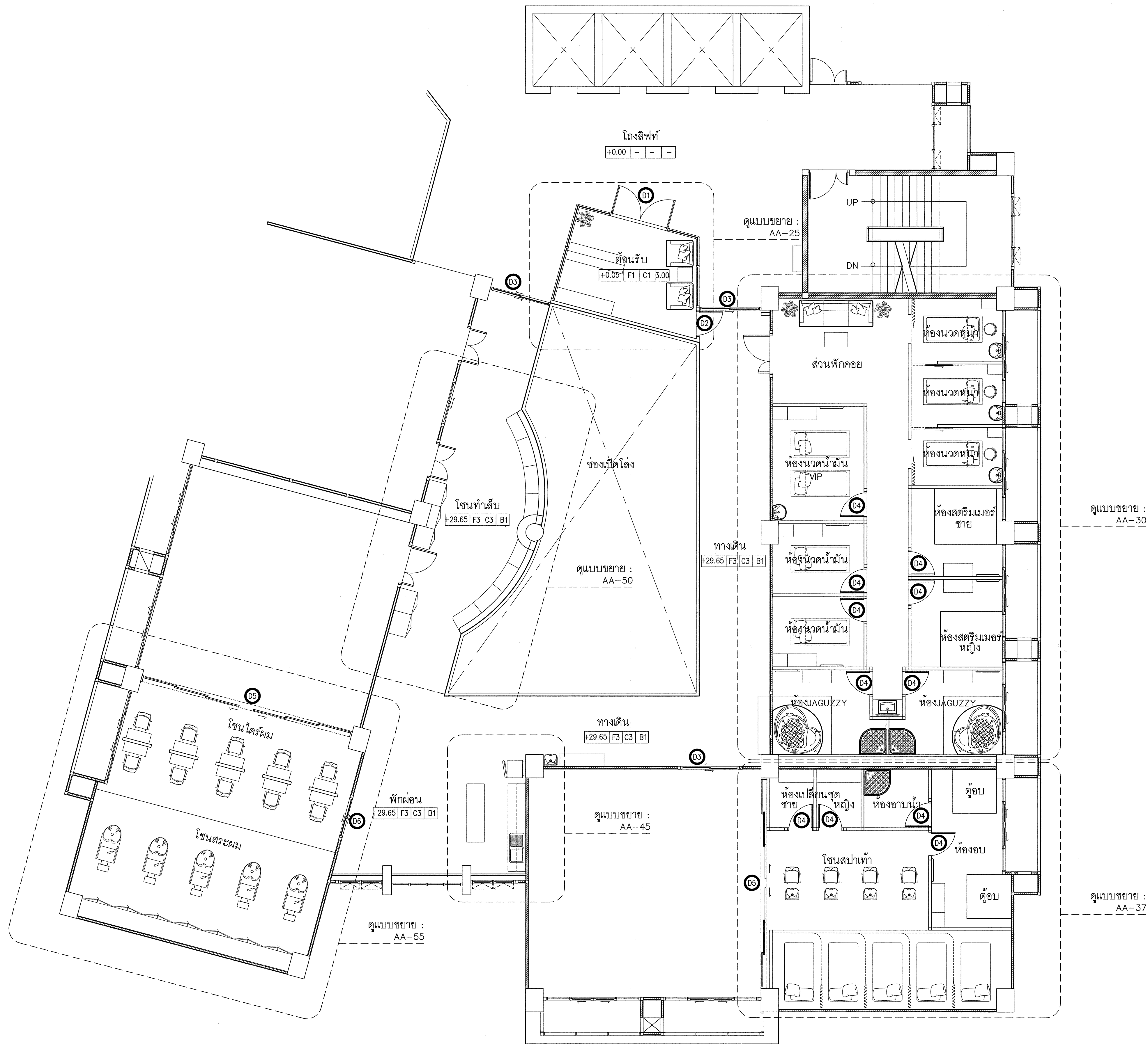
แปลนขยายแสดงพื้นที่งานตกแต่งชั้น 8 มาตราส่วน 1:75
