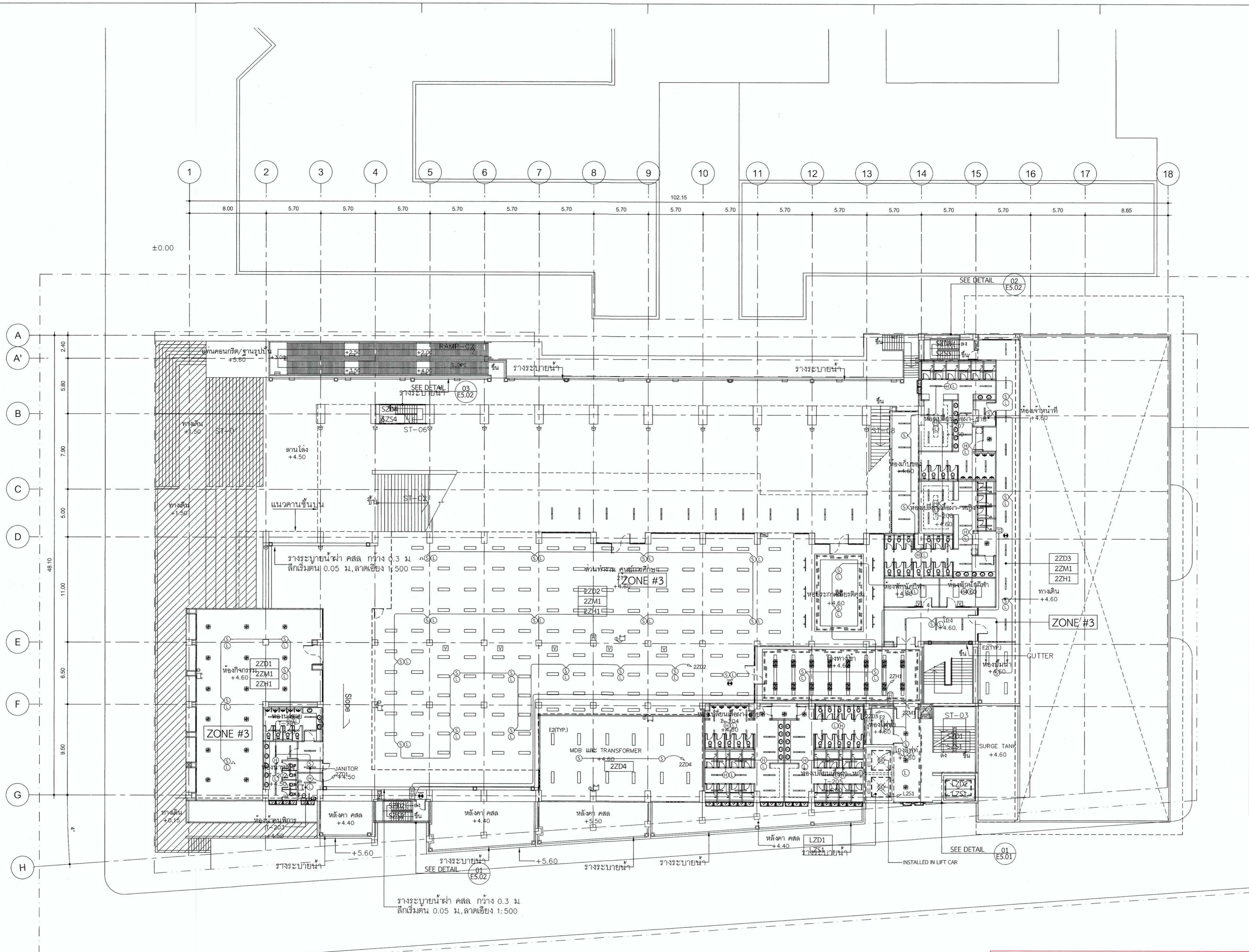
ผังระบบสัญญาณแจ้งเหตุเพลิงไหม้ ชั้นที่ 2 SCALE 1:200
