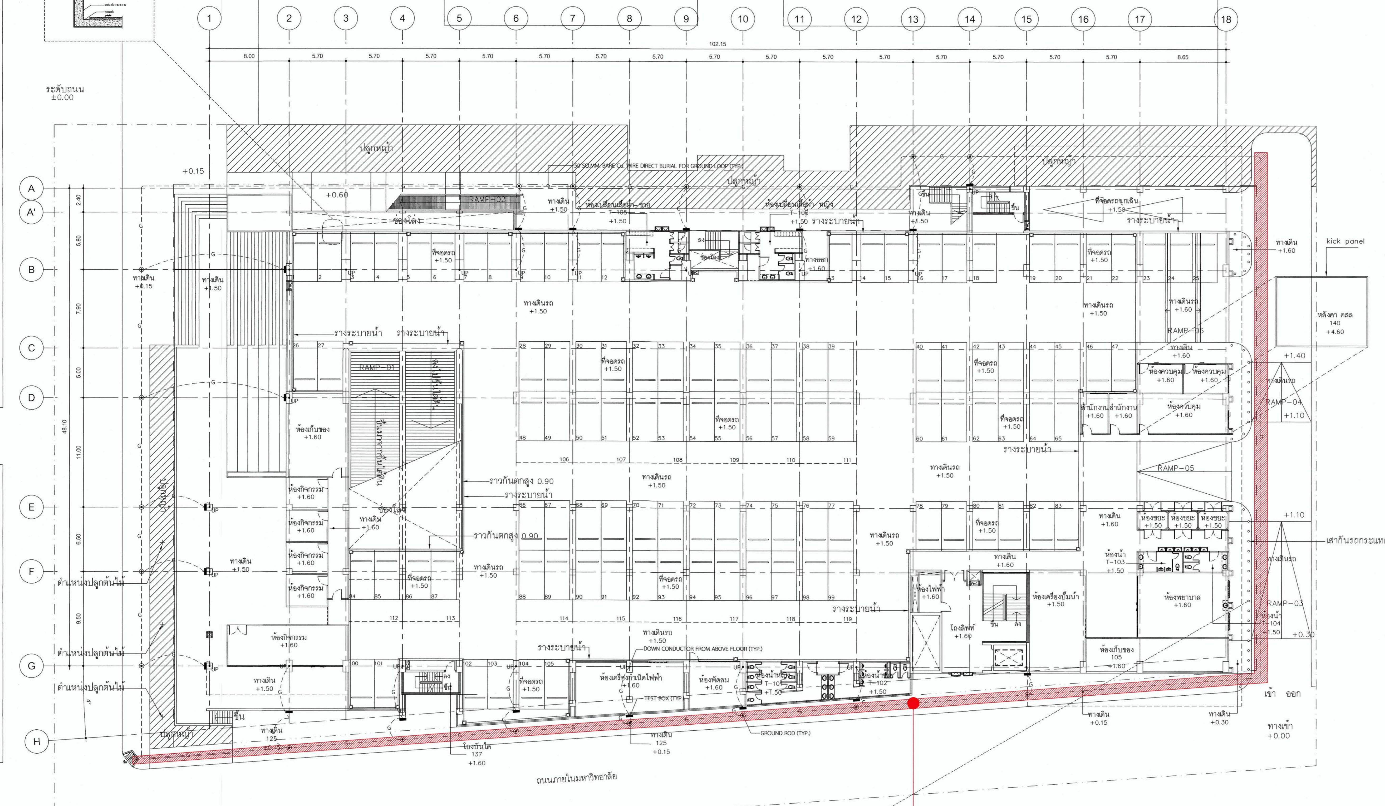
ผังระบบป้องกันฟ้าผ่าและการต่อลงดิน ชั้น 1 SCALE 1: 250
