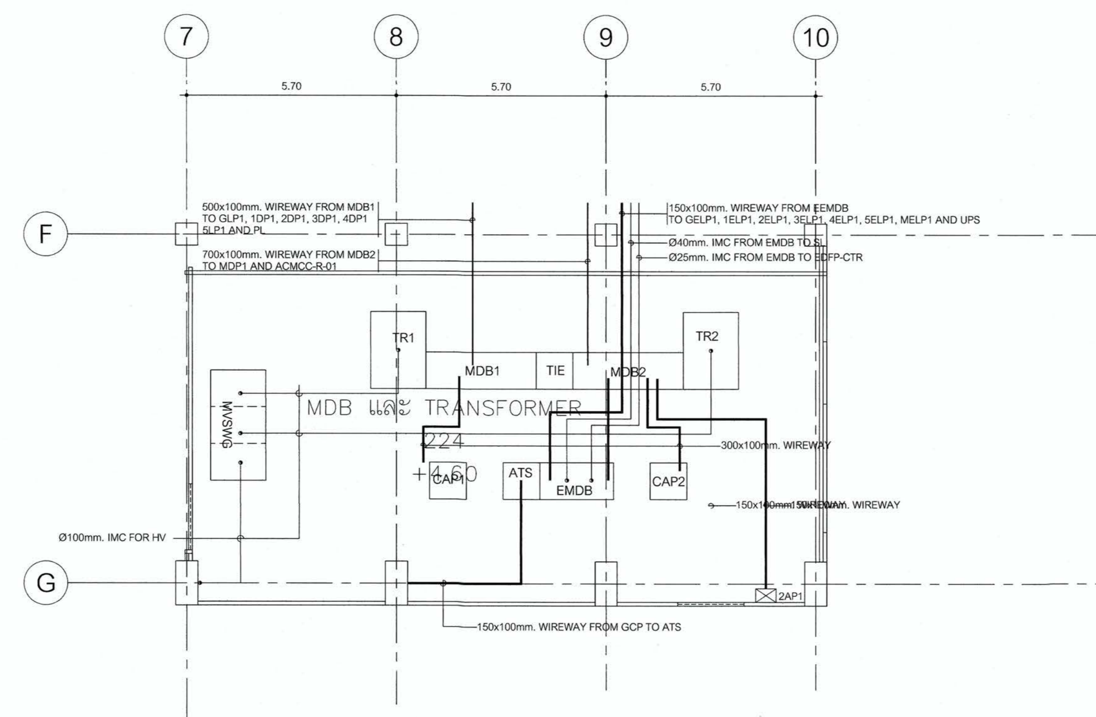
01 แบบขยายห้อง MDB
