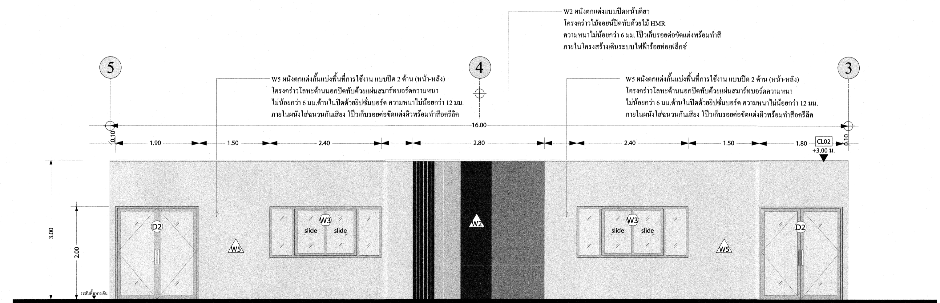
รูปด้านห้องปฐมพยาบาลหลังปรับปรุง SCALE 1:50
