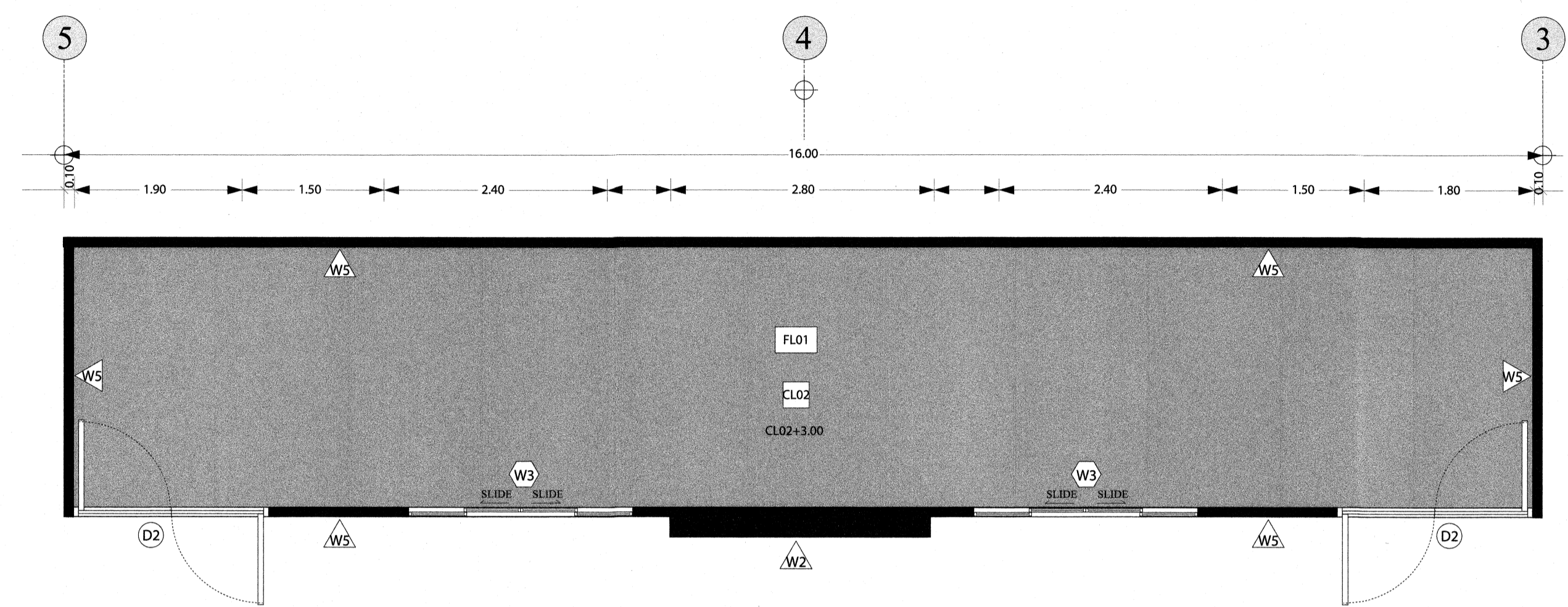
แบบขยายแปลนห้องปฐมพยาบาลหลังปรับปรุง SCALE 1:50
