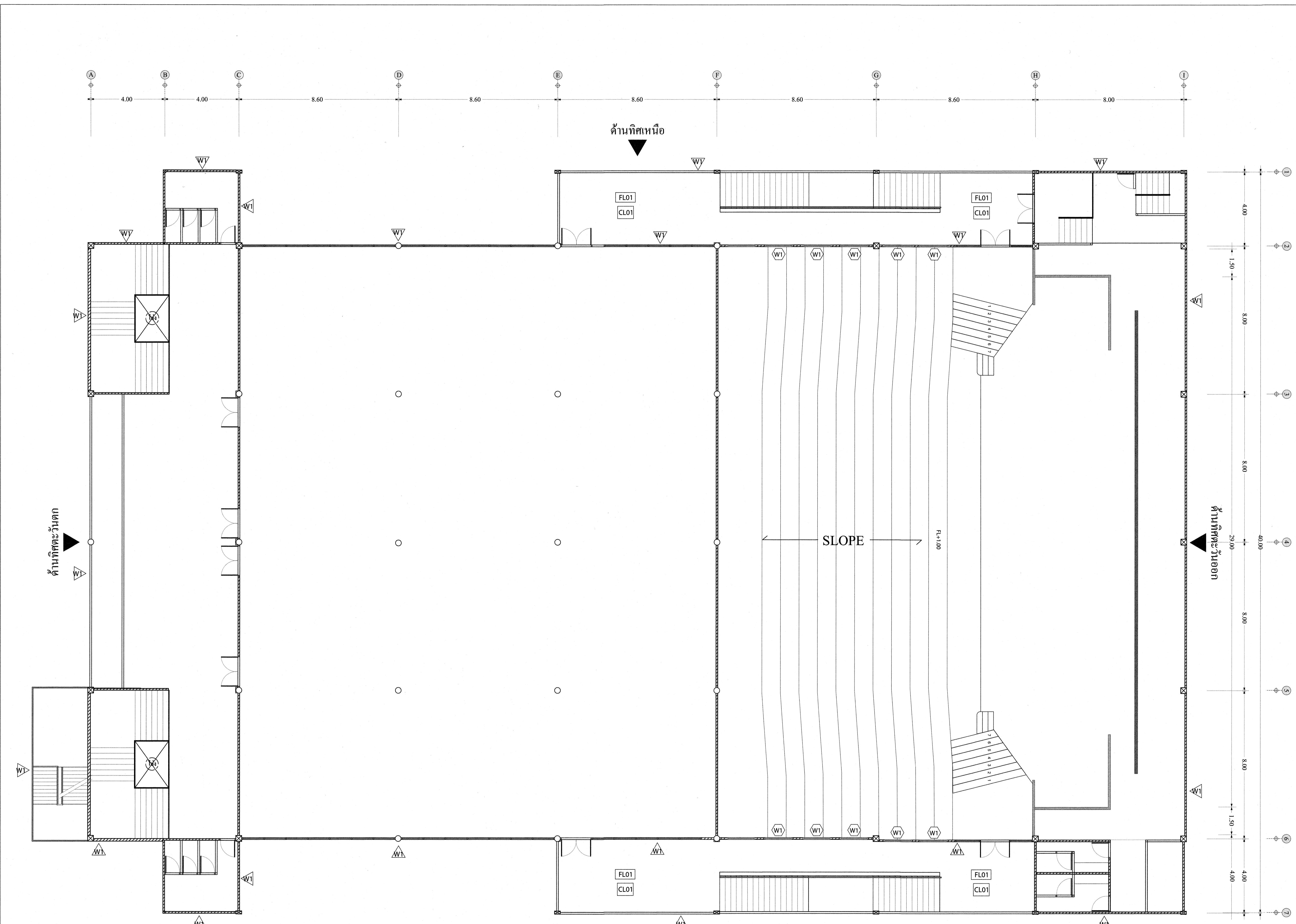
แปลนพื้นที่ 2 แบบปรับปรุง SCALE 1:100
