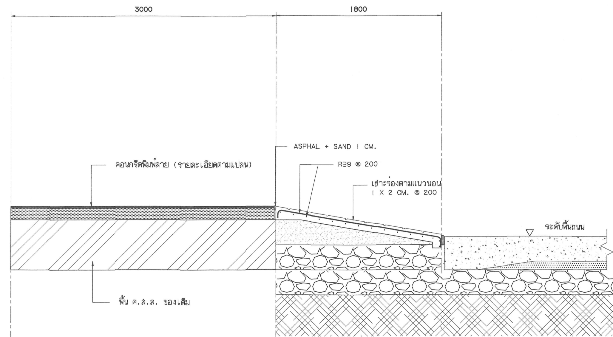
รูปตัดทั่วไปพื้นคอนกรีตพิมพ์ลาย
