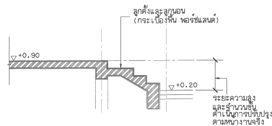
รูปตัดขยายบันได ด้านข้าง SCALE 1 : 50
