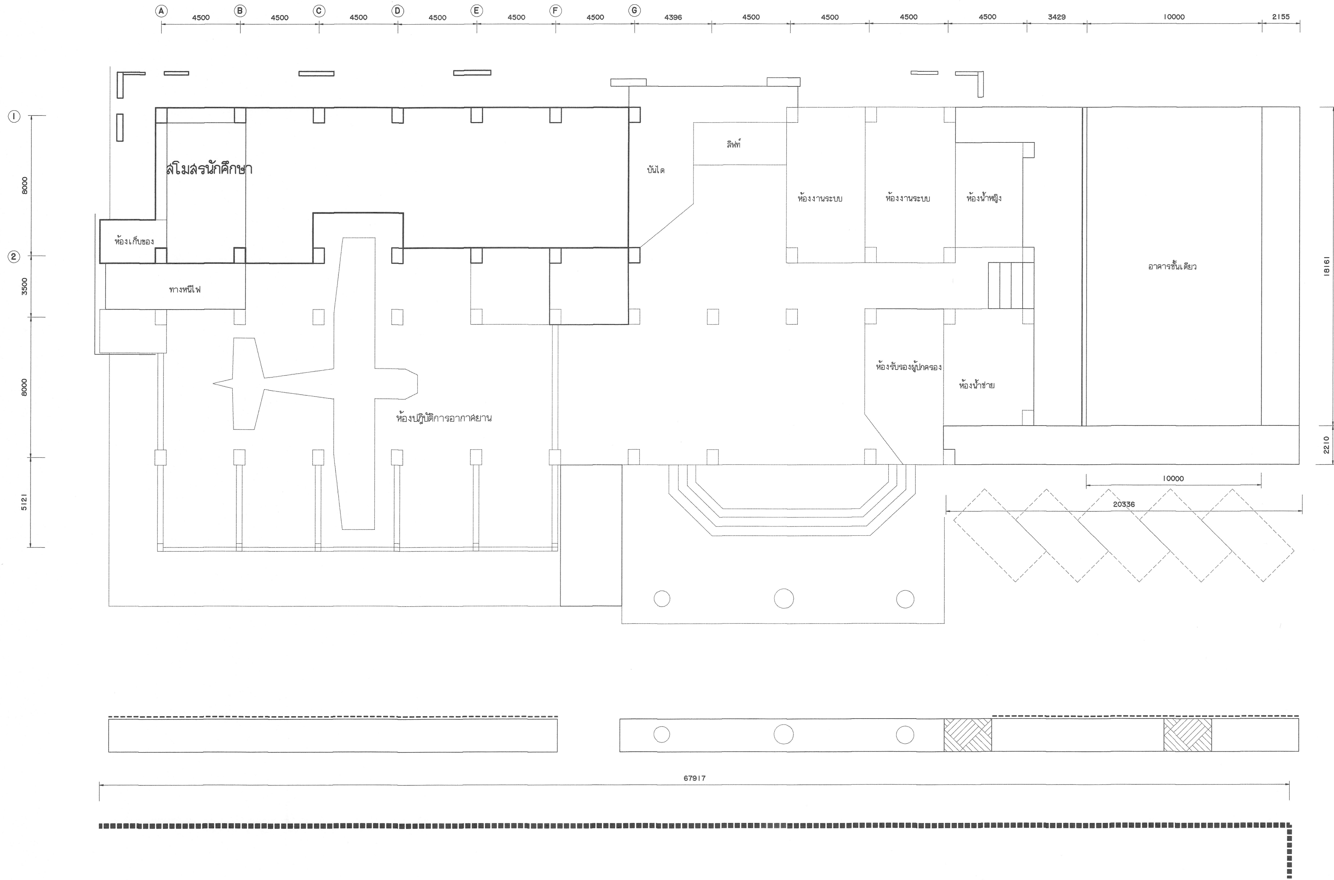
แปลนชั้นล่างอาคาร 48 คณะวิศวกรรมศาสตร์ มาตรฐาน 1 : 125 ก่อนปรับปรุง
