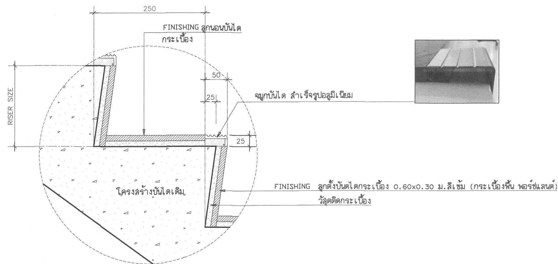
NOSING DETAIL N.T.S
