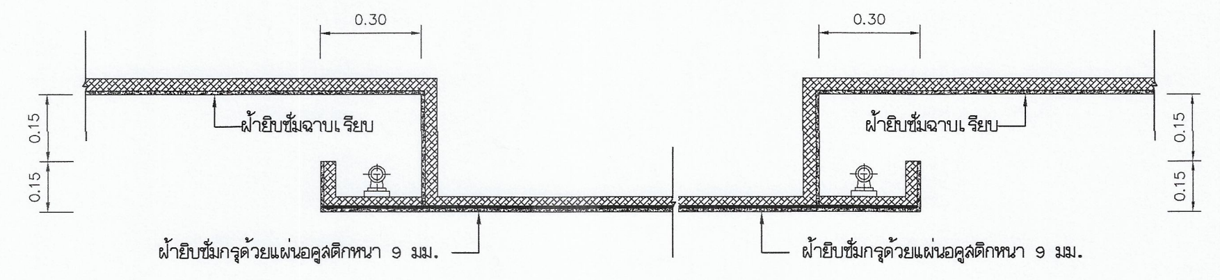
รูปตัด D Scale: 1:10
