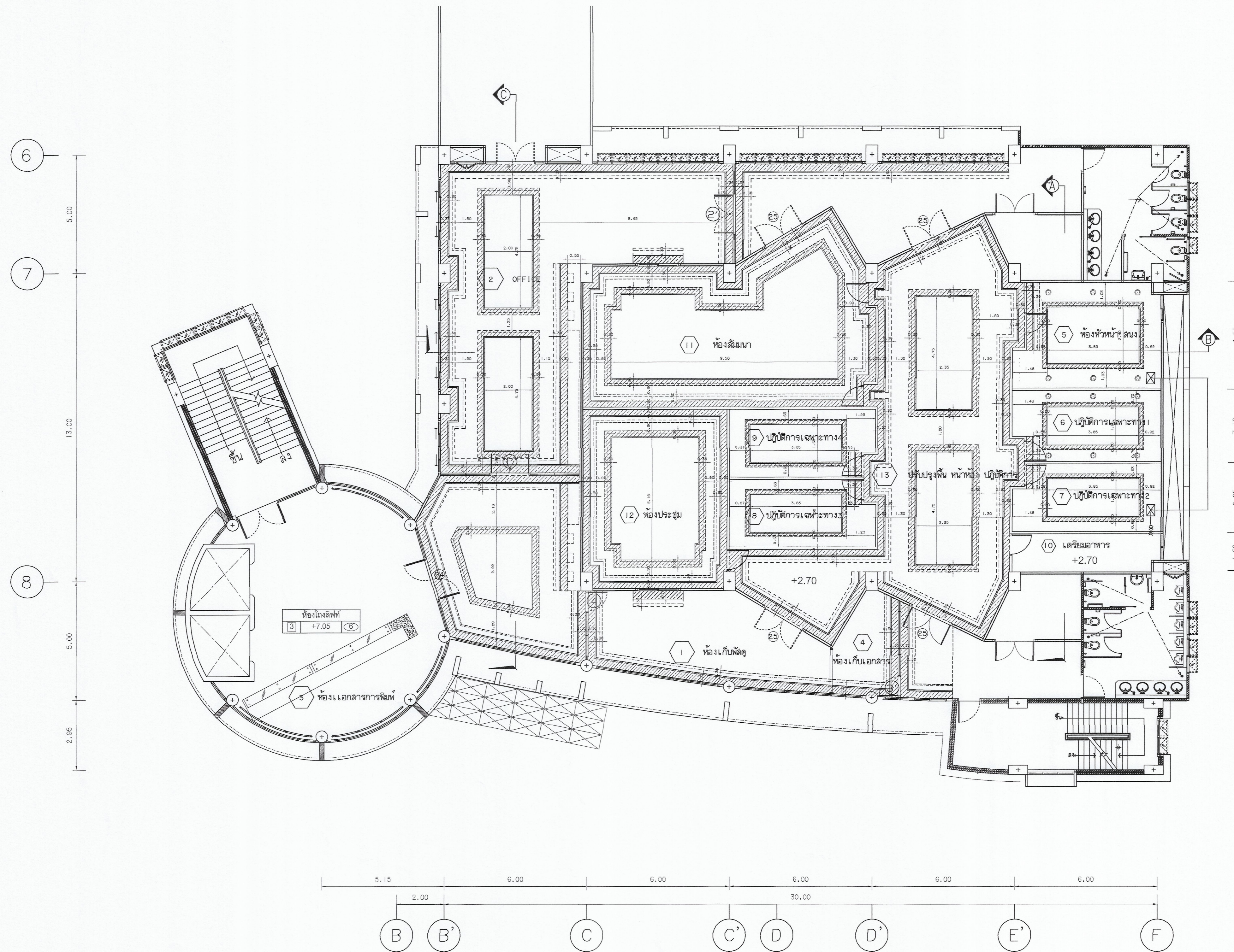
แปลนฝ้าเพดานชั้น 2 (2) ระดับ +7.05 (อาคารล่วงหน้า) มาตราส่วน 1 : 100
