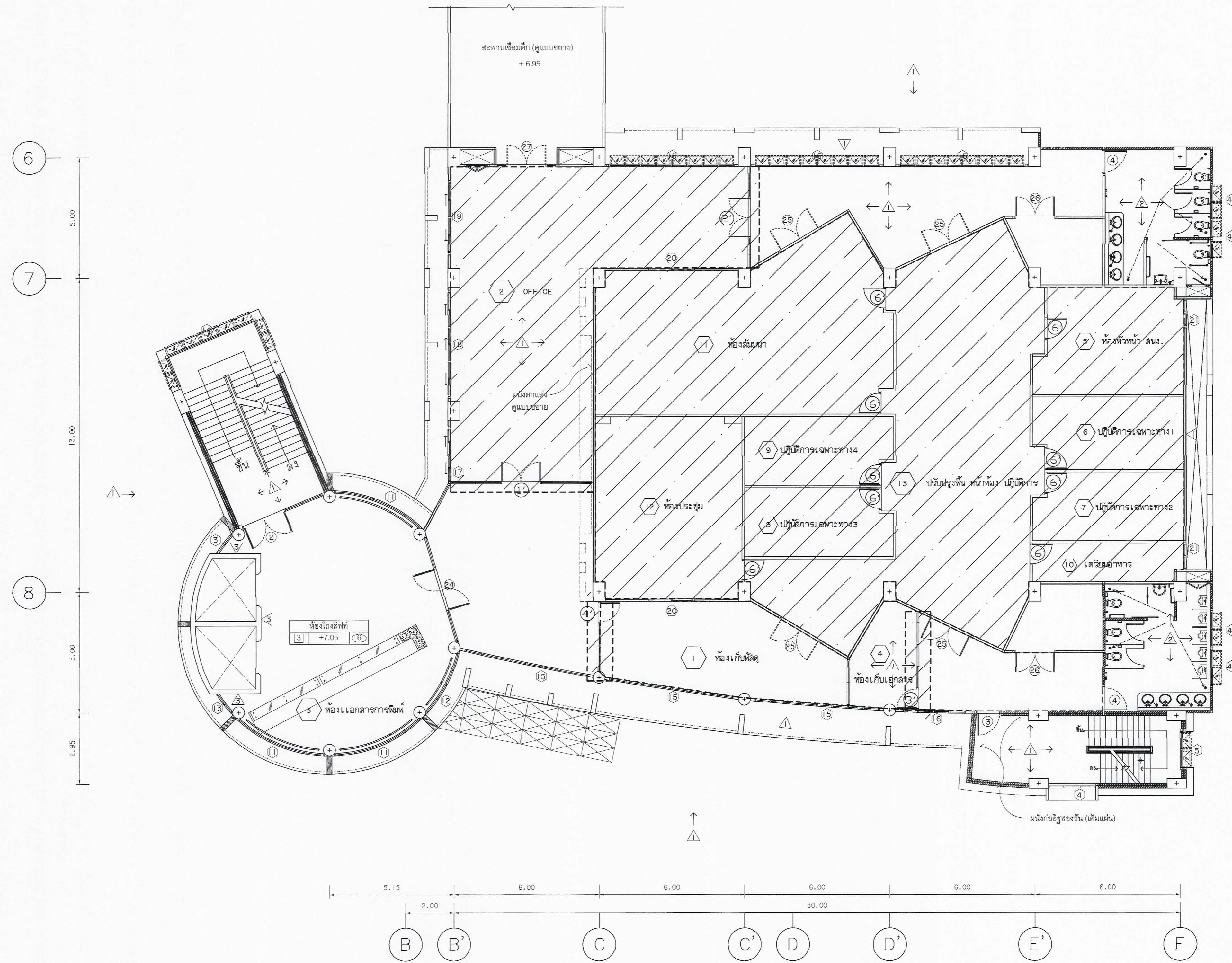
แปลนพื้นที่ 2 (อาคารส่วนหน้า) มาตราส่วน 1 : 100
