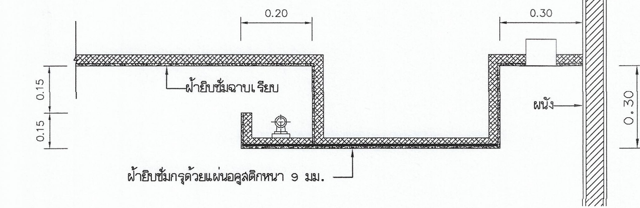
รูปตัด E Scale: 1:10
