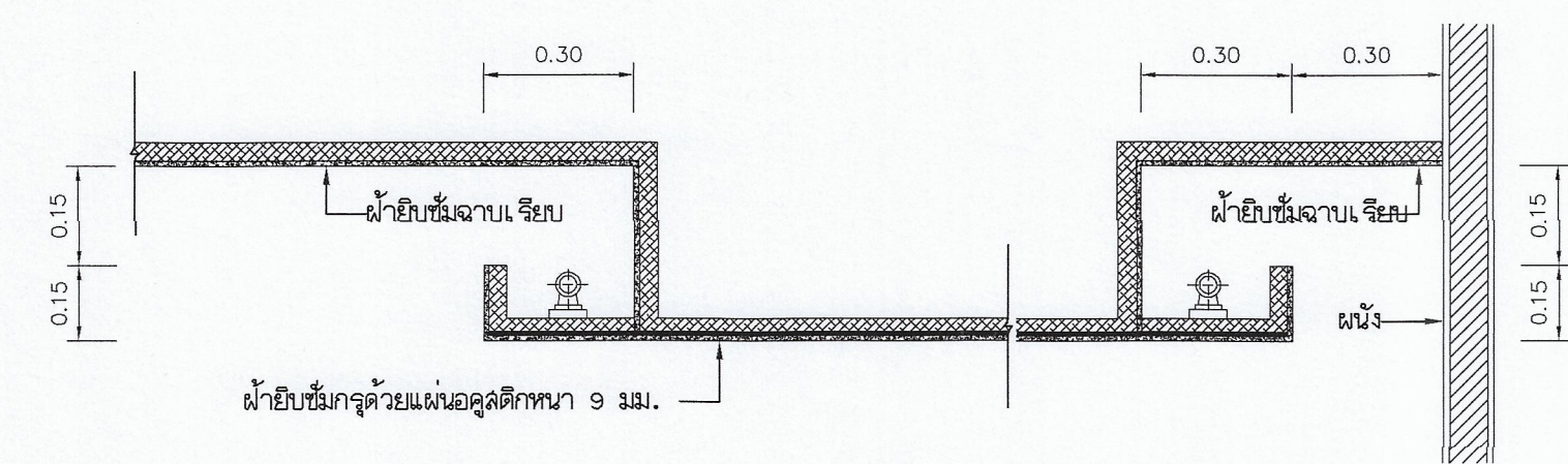
รูปตัด C Scale: 1:10
