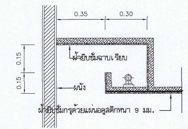
รูปตัด G Scale: 1:10
