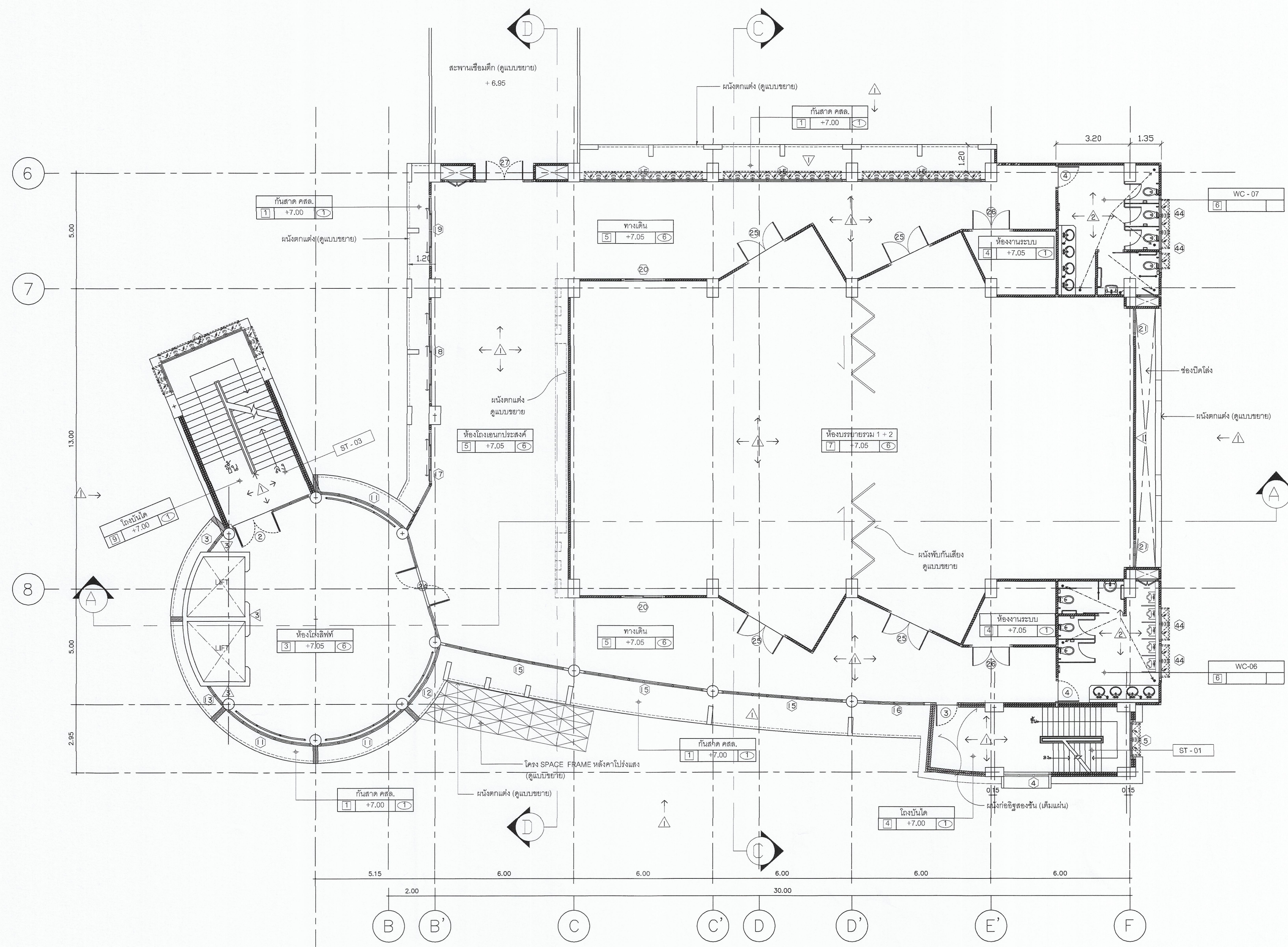
แปลนพื้นที่ชั้น 2 (อาคารส่วนหน้า) มาตราส่วน 1 : 100
