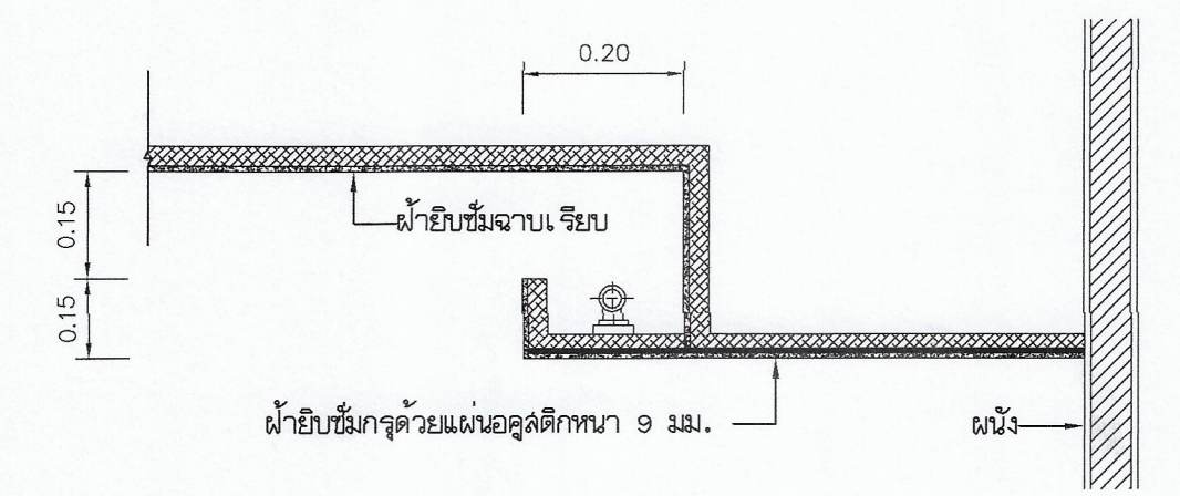
รูปตัด F Scale: 1:10
