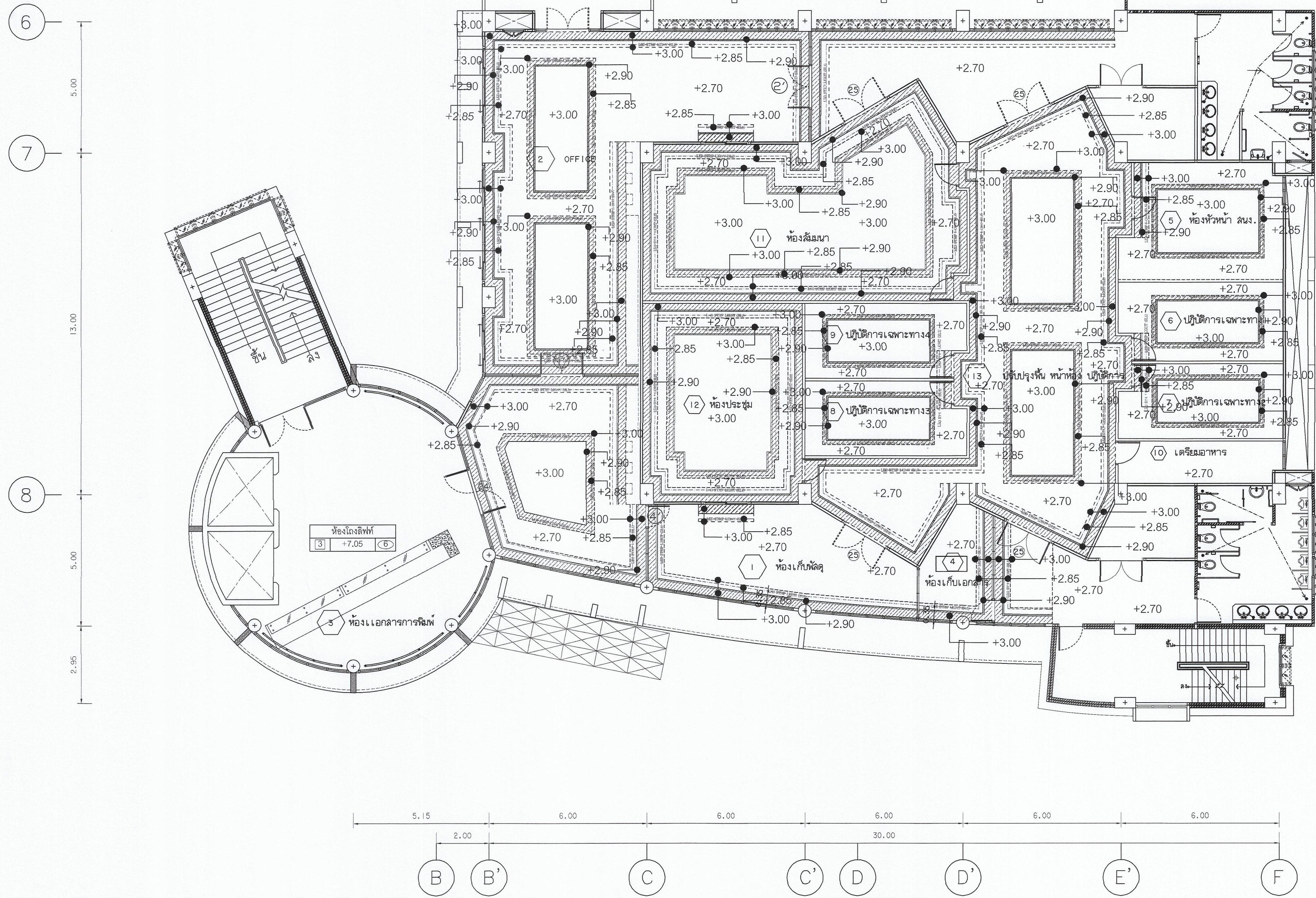
แปลนฝ้าเพดานชั้น 2 (1) ระดับ +7.05 (อาคารส่วนหน้า) มาตราส่วน 1:100
