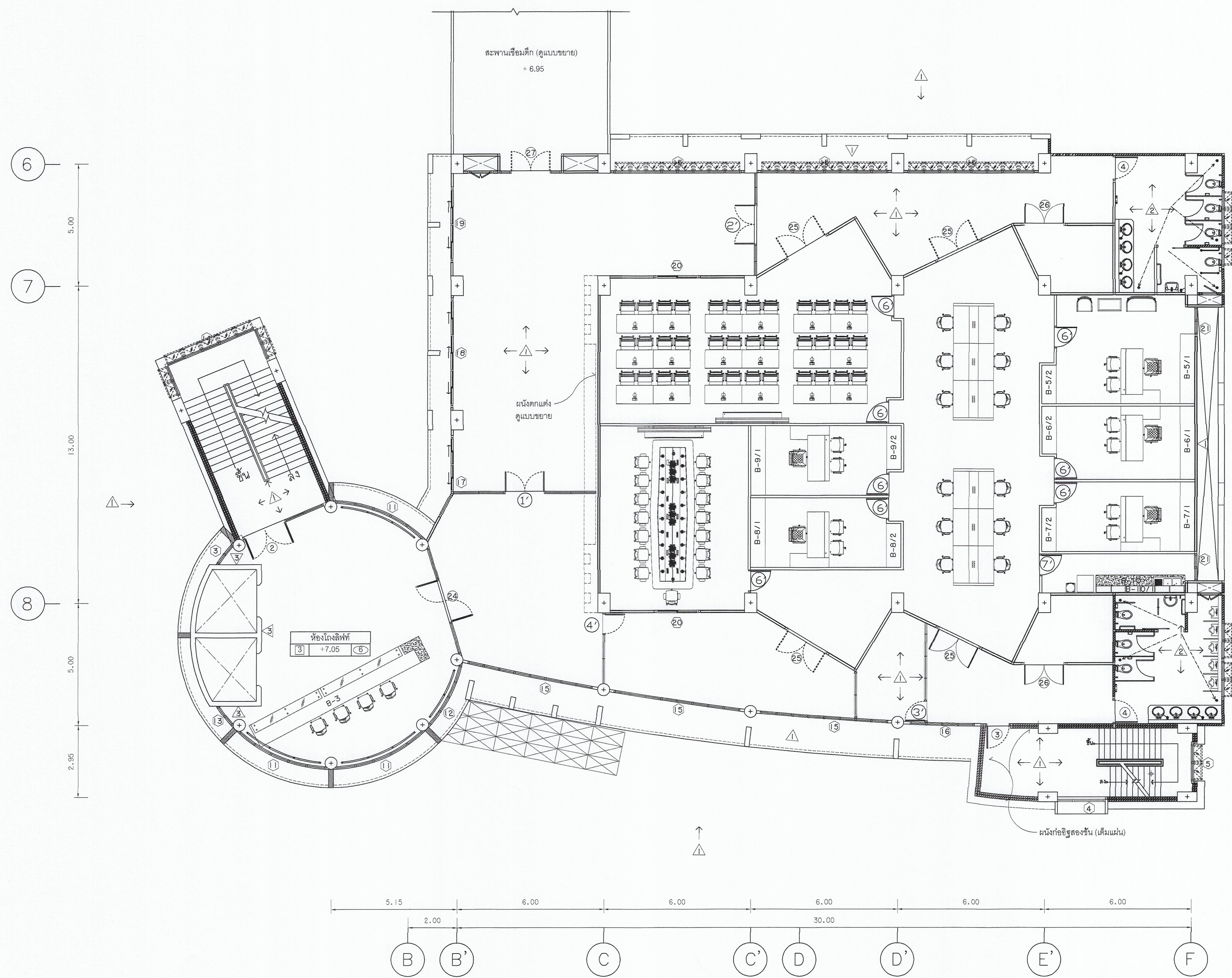
ผังเฟอร์นิเจอร์ชั้น 2 มาตรฐาน 1 : 100 หลังการปรับปรุง
