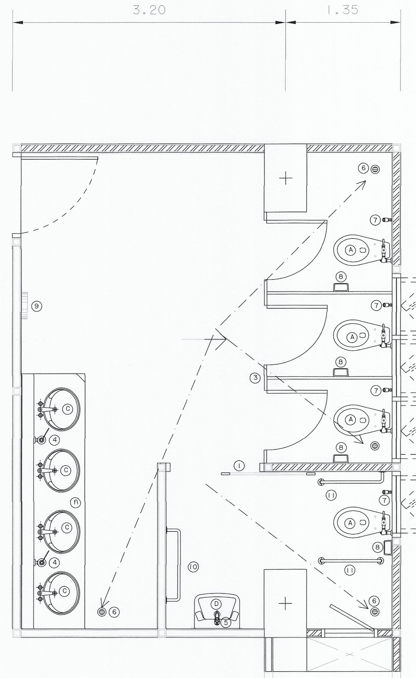
แปลนห้องน้ำหญิง มาตราส่วน 1 : 25
