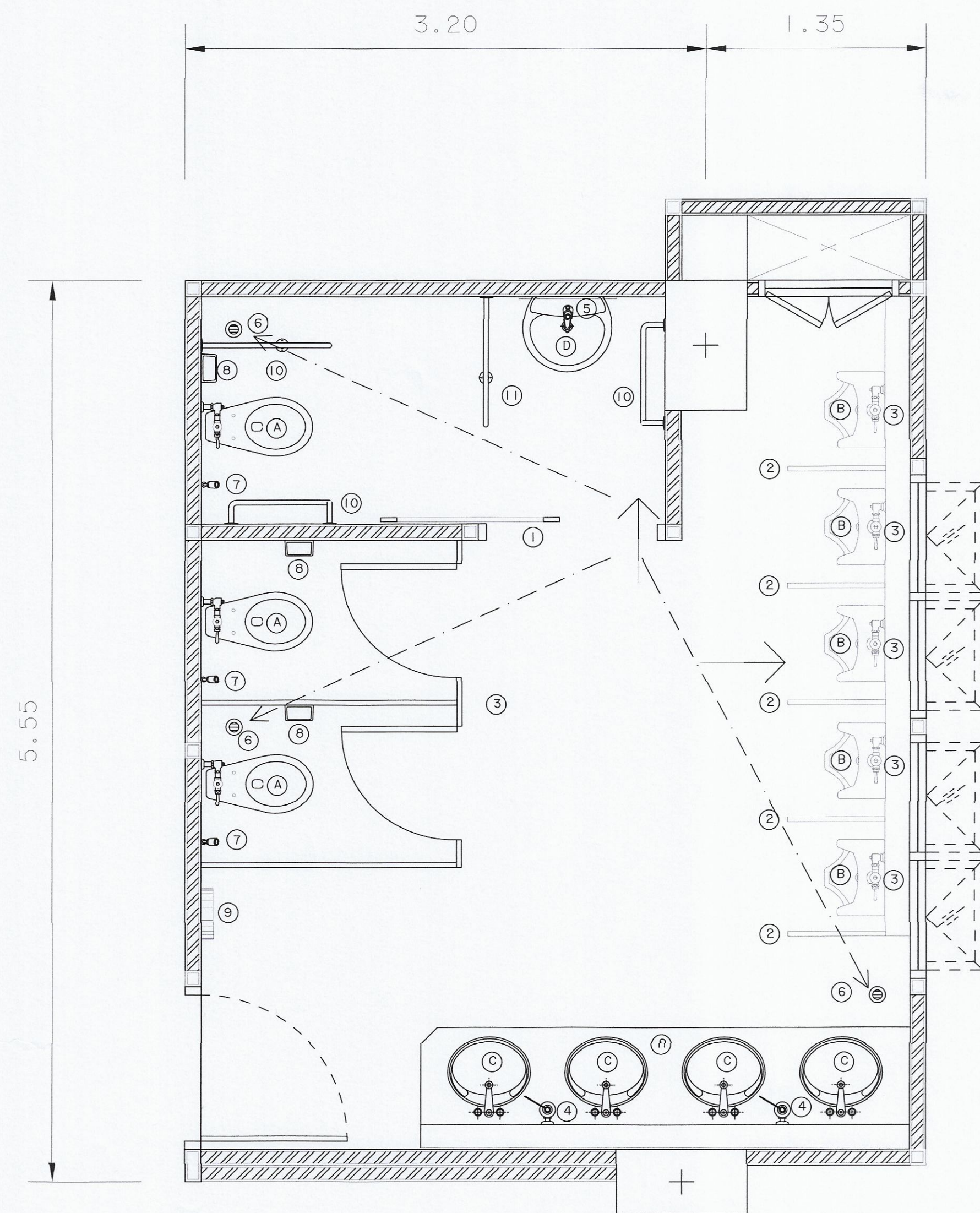
แปลนห้องน้ำชาย มาตราส่วน 1 : 25
