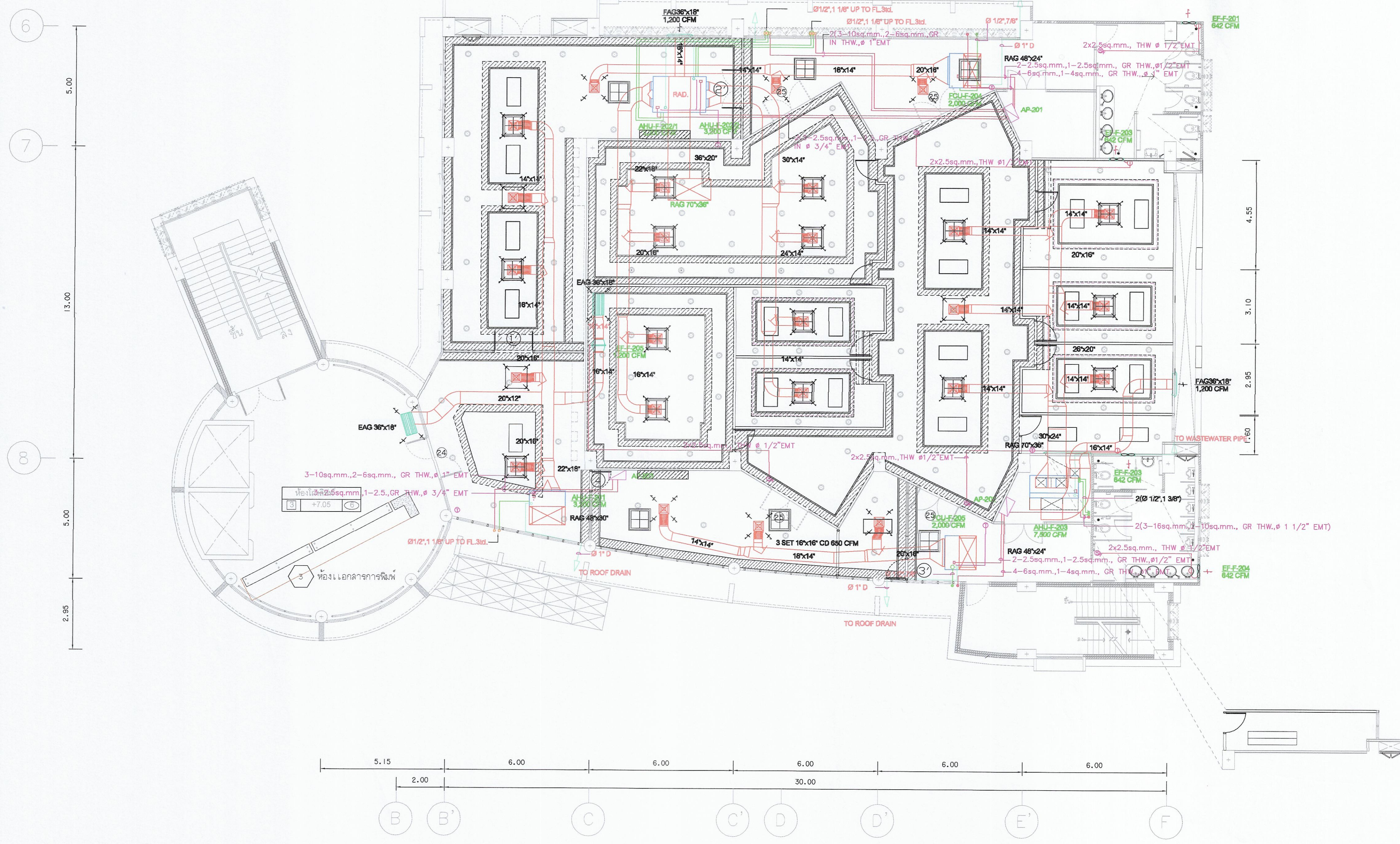
แปลนระบบปรับอากาศ และระบายอากาศ ระดับ +7.05 (อาคารส่วนหน้า) 1:100
