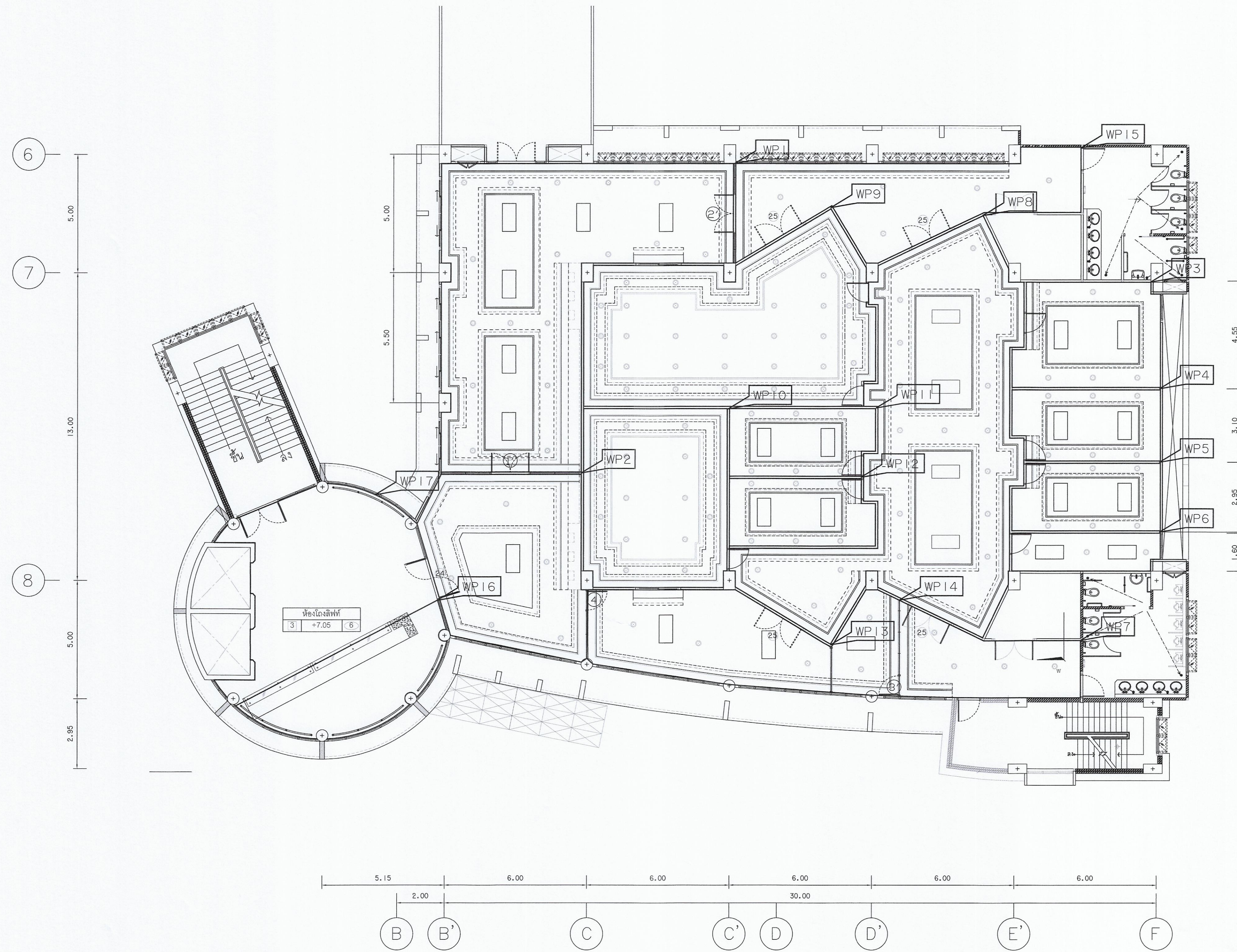
แปลนระบบไฟฟ้าส่องสว่างชั้น 2 ระดับ +7.05 (อาคารส่วนหน้า)
