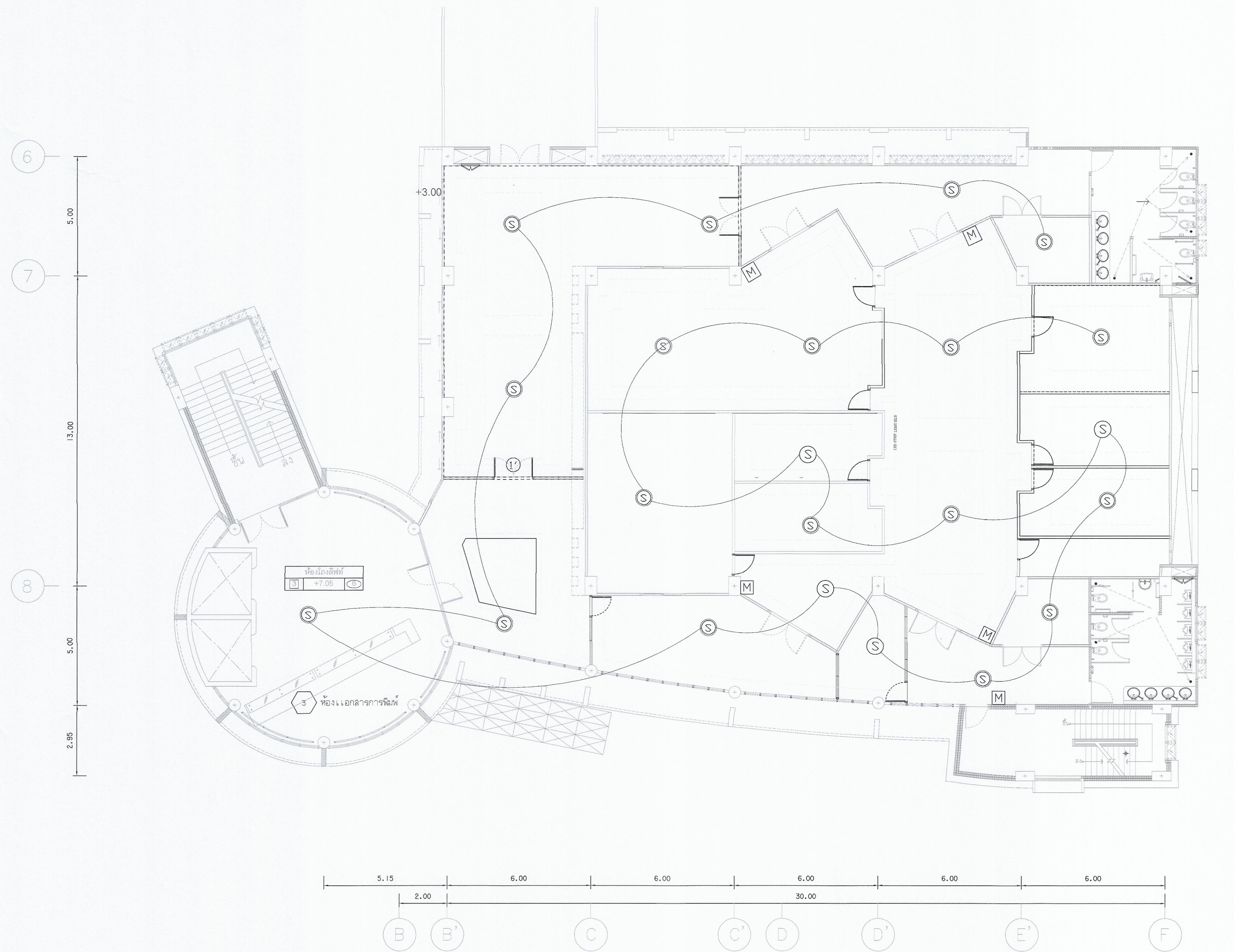
แปลนระบบไฟฟ้าส่องสว่างชั้น 2 ระดับ +7.05 (อาคารส่วนหน้า) มาตรฐาน 1:100
