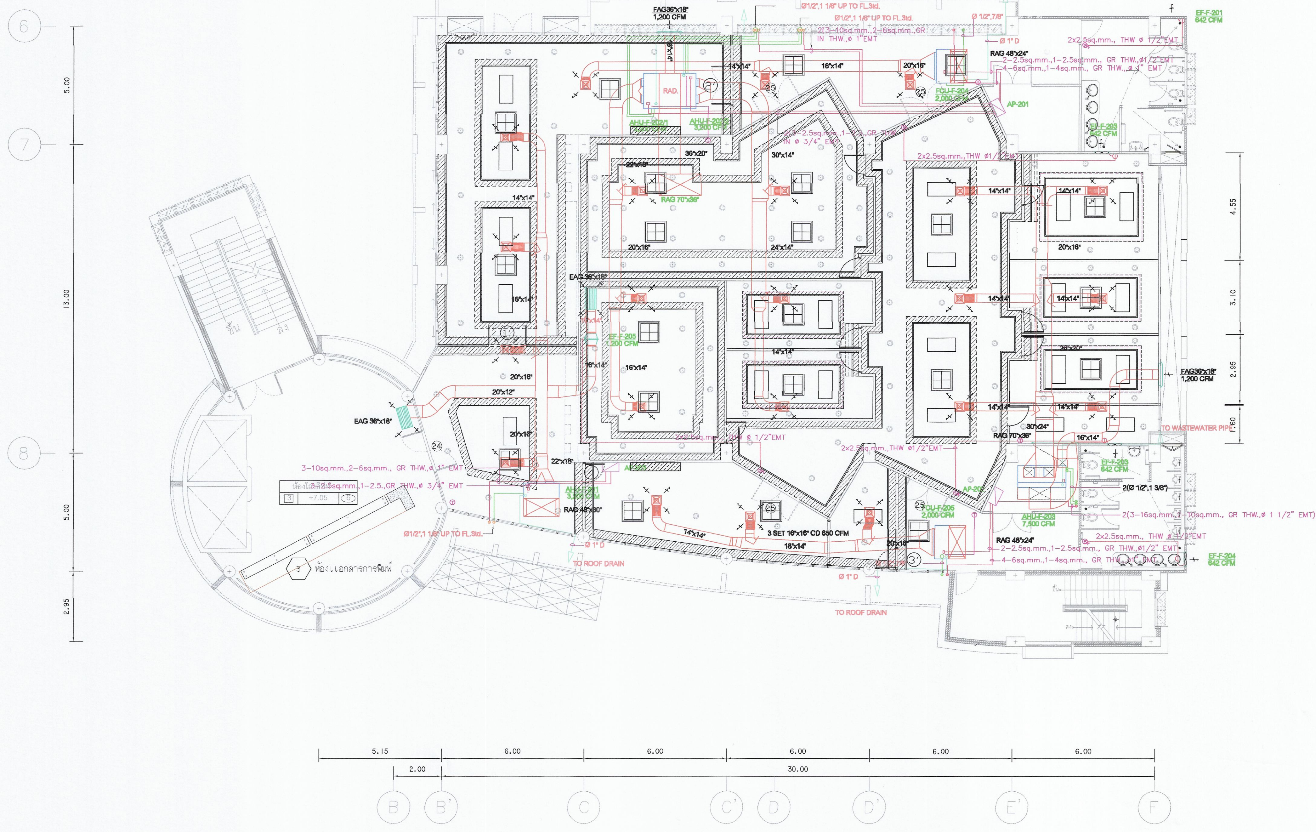
แปลนระบบปรับอากาศ และระบายอากาศ ระดับ +7.05 (อาคารส่วนหน้า) มาตราส่วน 1:100
