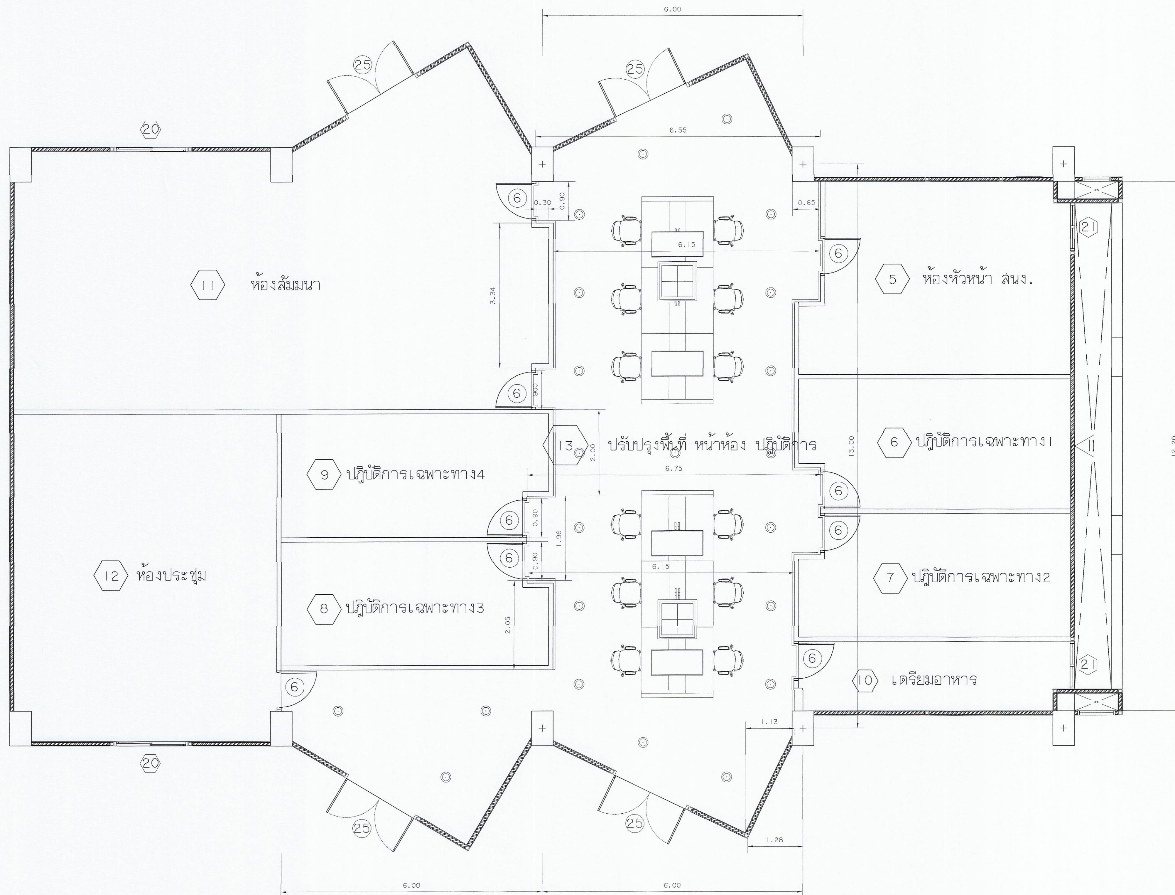
แปลนปรับปรุงพื้นที่ หน้าห้อง ปฏิบัติการ มาตราส่วน 1:50
