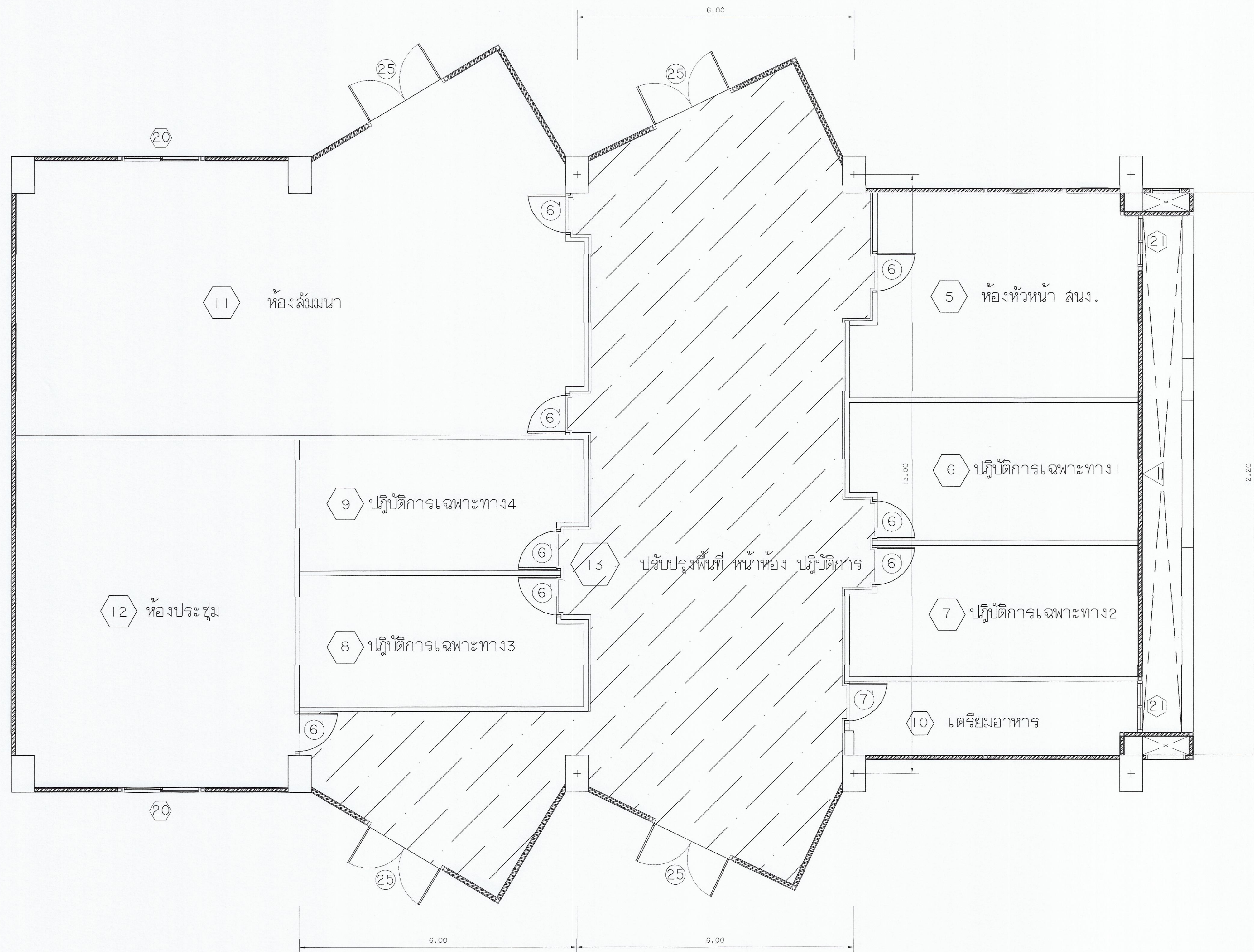
แปลนปรับปรุงพื้นที่ หน้าห้อง ปฏิบัติการ มาตราส่วน 1:50
