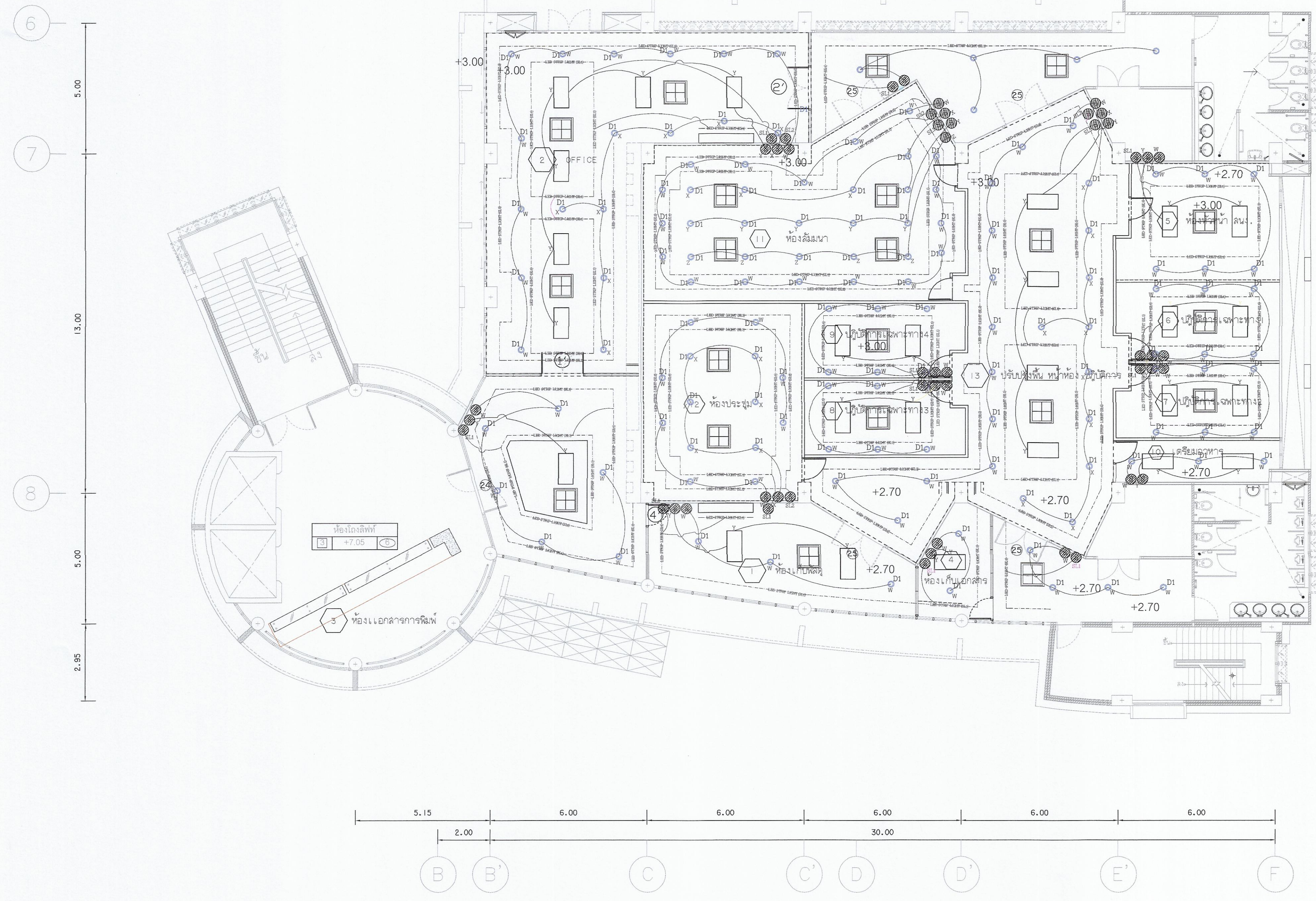
แปลนระบบไฟฟ้าส่องสว่างชั้น 2 ระดับ +7.05 (อาคารส่วนหน้า) มาตรฐาน 1 : 100
