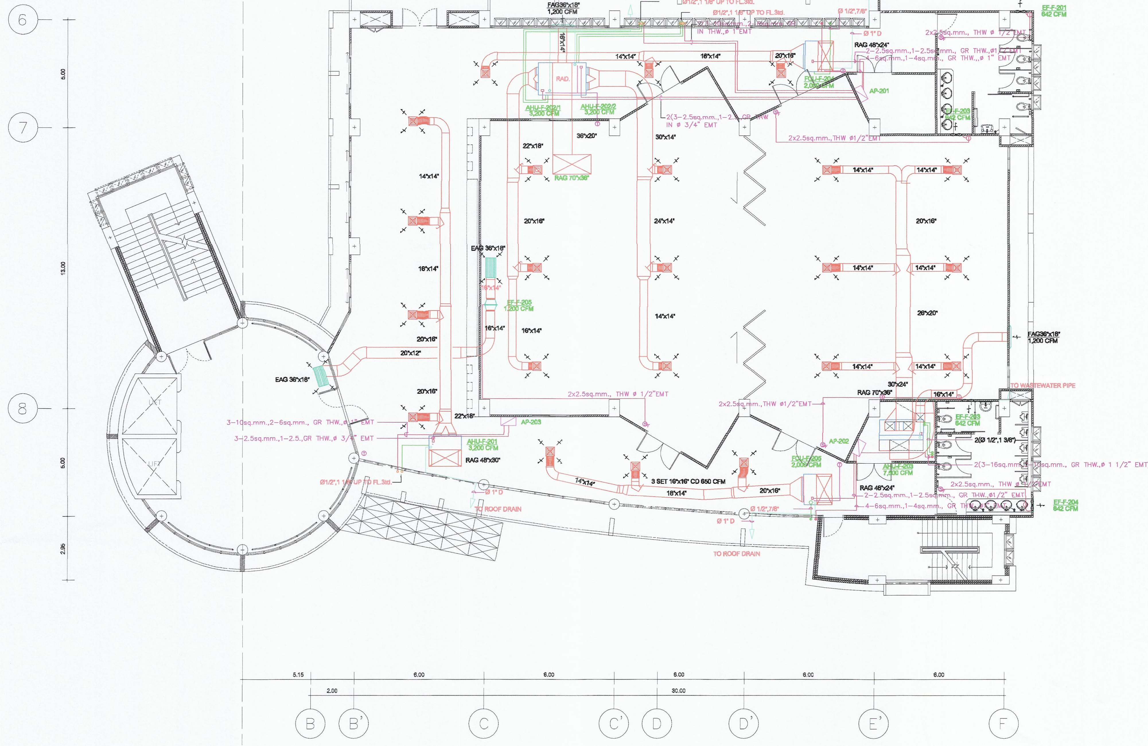
แปลนระบบปรับอากาศ และระบายอากาศ ระดับ +7.05 (อาคารส่วนหน้า) มาตรฐาน 1:100
